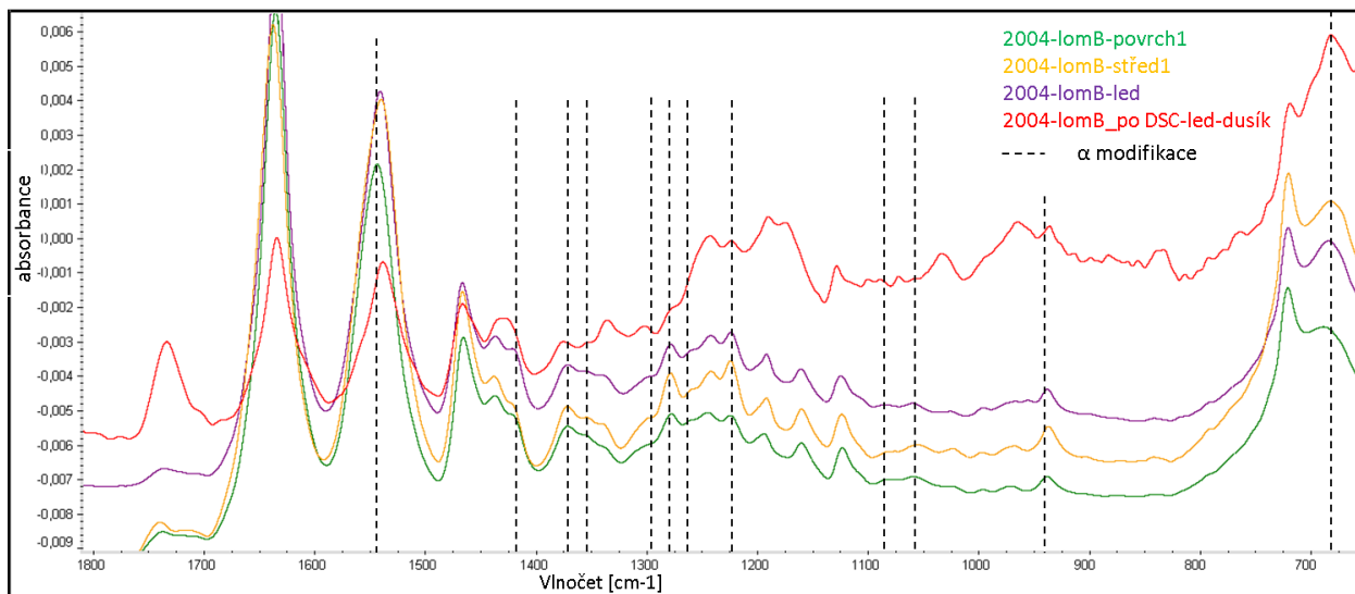
Obr 14: FTIR-ATR spektra spony 2004-lomB-povrch1 (zelená), 2004-lomB-střed1 (žlutá) a materiálu spon roztavených a následně a zchlazených ve směsi vody a ledu a znovu v kapalném dusíku:
