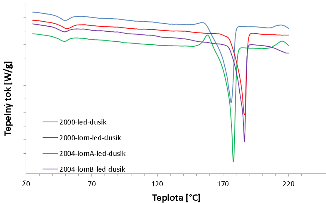
Obr 10: Endotermické křivky prvního ohřevu chlazených vzorků spon 2000, a 2004; exo děje nahoru; hlavní jednotka osy y odpovídá 0,2 W/g
