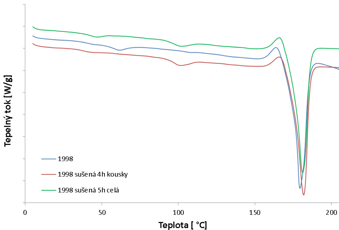
Obr. 9: Endotermické křivky prvního ohřevu sušené a nesusušené spony 1998, exo děje nahoru; hlavní jednotka osy y odpovídá 0,2 W/g
