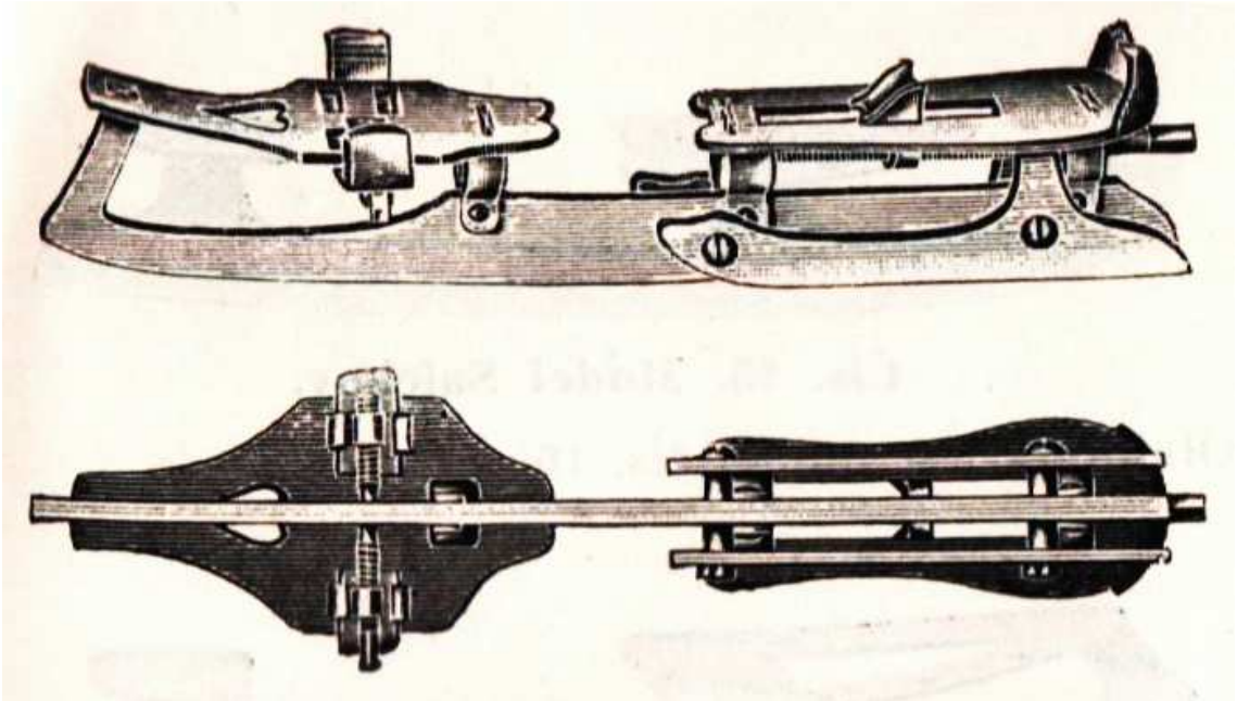
Obrázek č. 19 Brusle s opěrnými želízky – model Hercules Primus*
