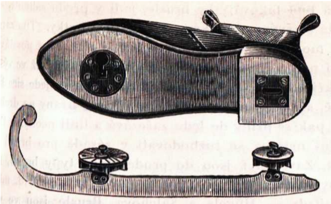
Obrázek č. 20 Ukázka připevnění brusle k botě*
