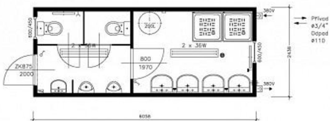
Obrázek 15: Sanitární kontejner
