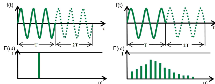
Obrázok 3.2: Presakovanie spektra
