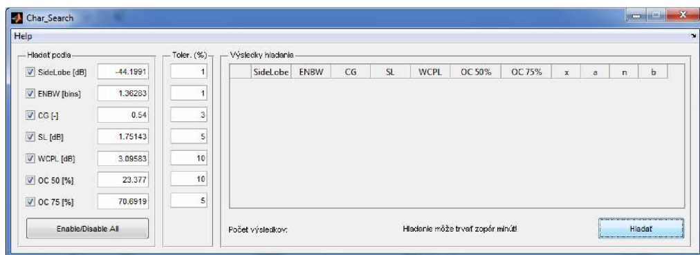
Obrázok 3: Napodobňovanie okna Hamming
