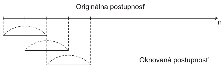
Obrázok 4.5: Rozloženie postupnosti pre spracovanie s prekrytím
