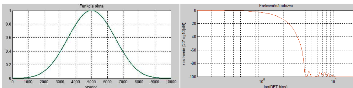
Obrázok 3.9: Blackman-Harris okno a jeho frekvenčná odozva
