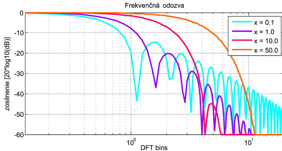
Obrázok 6.3: Frekvenčné odozvy parametrizovaného okna s parametrom „x“
