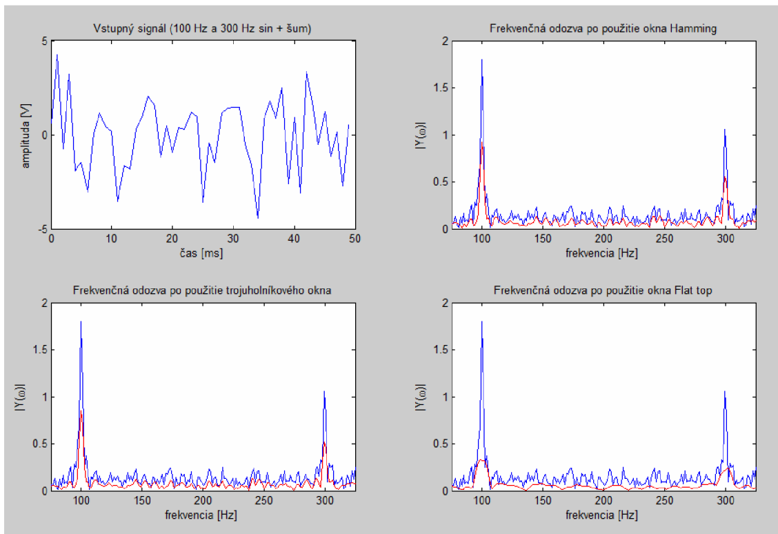
Obrázok 5.1: Príklad na chovanie sa frekvenčnej odozvy pri použití časových okien trojuholník, Hamming a Flat top
