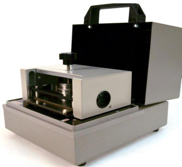
Obr. 27: Třielektrokový měřicí systém Agilent 16008B Resistivity Cell, upraveno podle [19]
