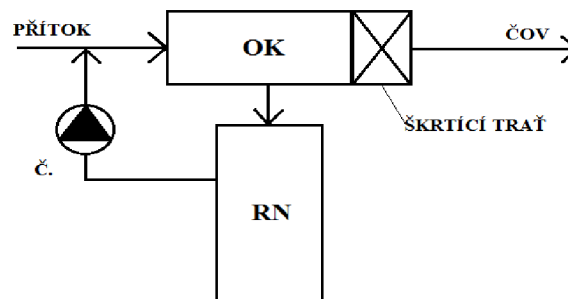
Obr. 4.2 - Příklad zapojení dešťové nádrže do stokové sítě ve vedlejší směru [4]
