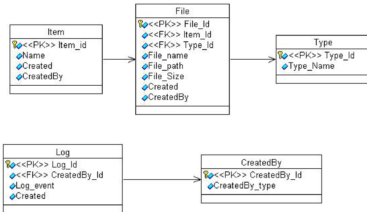
Obrázek 5-1: Diagram tříd
