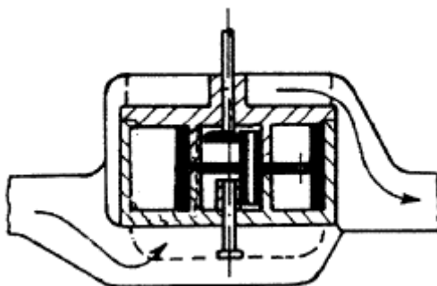
Obr. 5 – Řez vodoměru s krouživým pístem [2]
