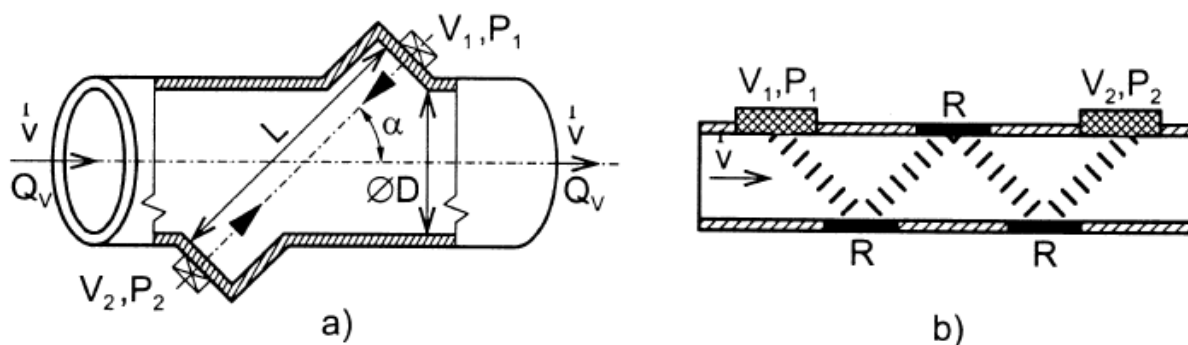
Obr. 8 – Ultrazvukové senzory průtoku a) V_1, V_2 je označení pro vysílači a P_1, P_2 přijímači funkci měnič, b) prodloužení ultrazvukového signálu reflektory R [9]
