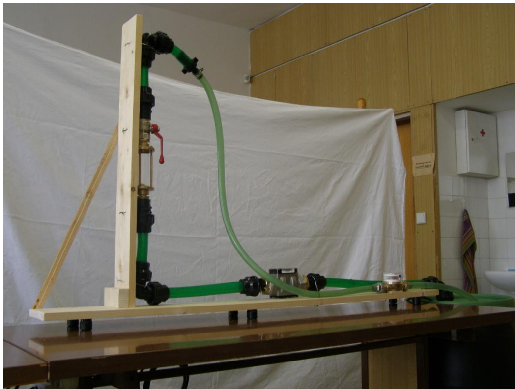
Obr. 12 – Nosná konstrukce
