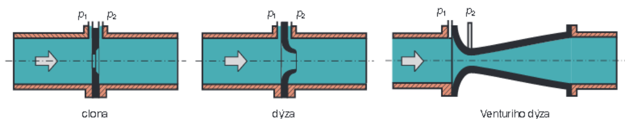
Obr. 3 – Škrtící orgány [3]
