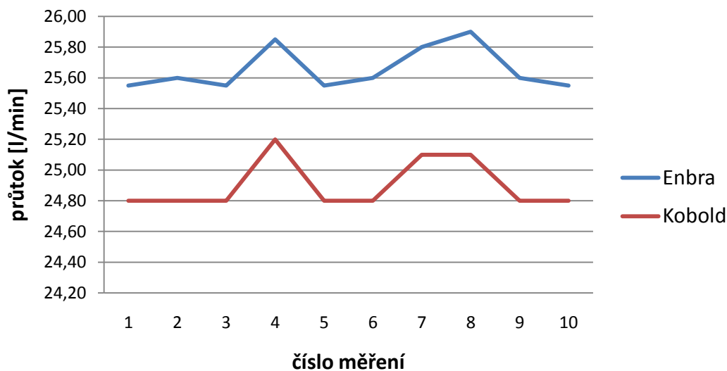
Graf 3 – průběh protékého množství s přiškrceným ventilem naměřené průtokoměry
