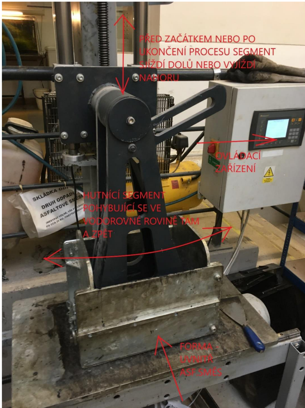
Obrázek 25 Ukázka segmentového zhutňovače [20]
