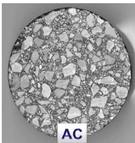
Obrázek 23 Jádrový vývrt asfaltového betonu [26]
