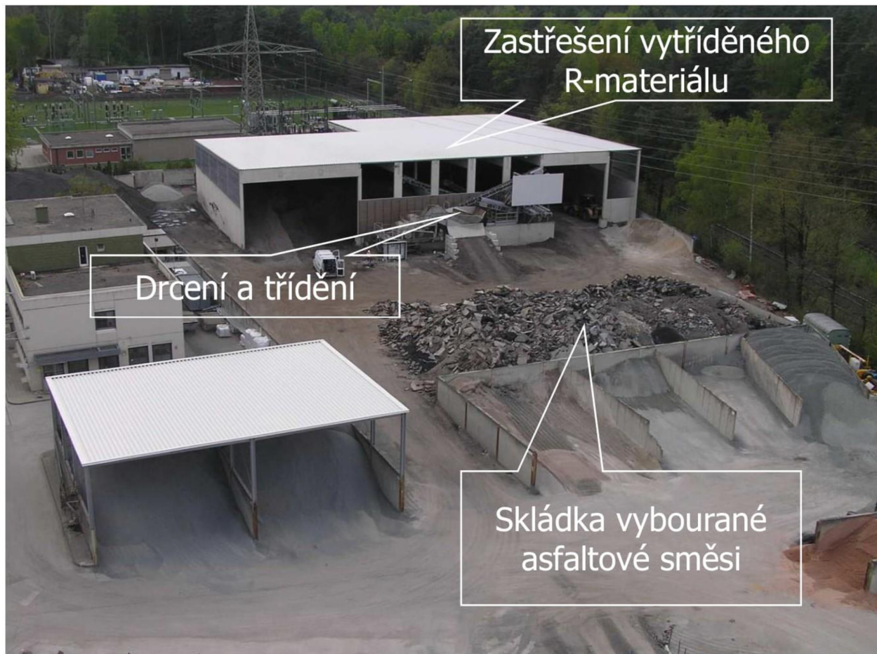
Obrázek 4 Skladování R-materiálu, drcení a třídění, zastřešení R-materiálu [9]
