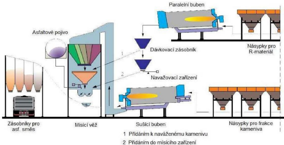
Obrázek 5 Přeohřívání R-materiálu v paralelním bubnu [9]
