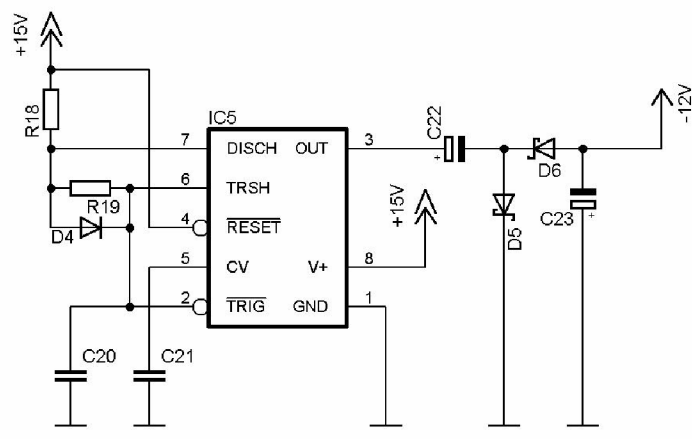
Obr. 12 Zapojení pomocného zdroje záporného napětí
