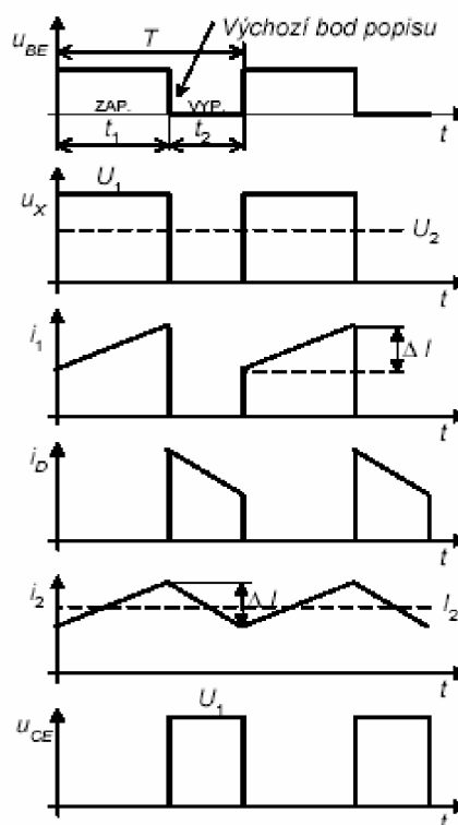
Obr. 7 Průběhy napětí a proudů na prvcích měniče [1]
