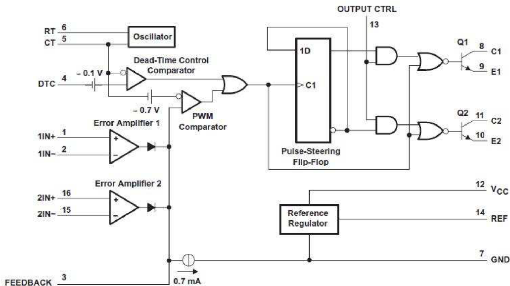
Obr. 9 Blokové schéma řídicího obvodu TL494 [3]
