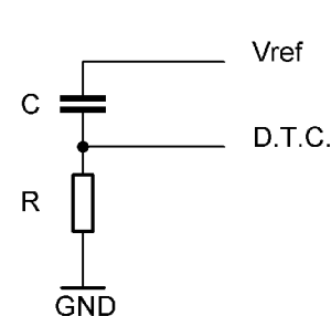
Obr. 10 Soft-start obvod
