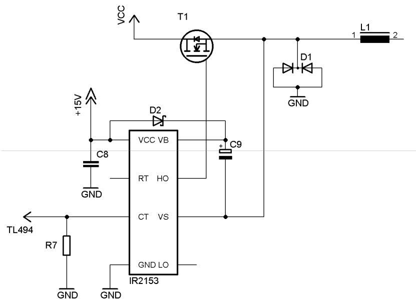
Obr. 11 Budič a výkonový obvod měniče
