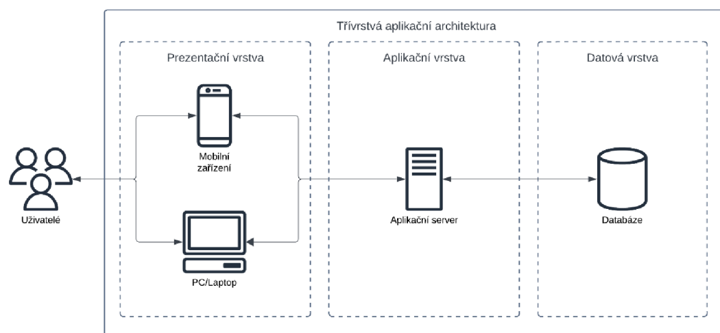
Obrázek 1: Vizualizace třívrstvé aplikační architektury
