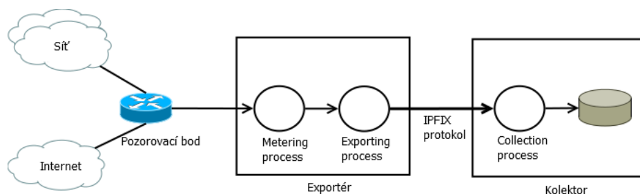
Obrázek 3.1: Jednoduchá architektura
