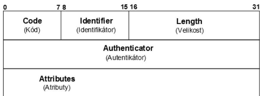
Obrázek 2.1: Formát RADIUS paketu
