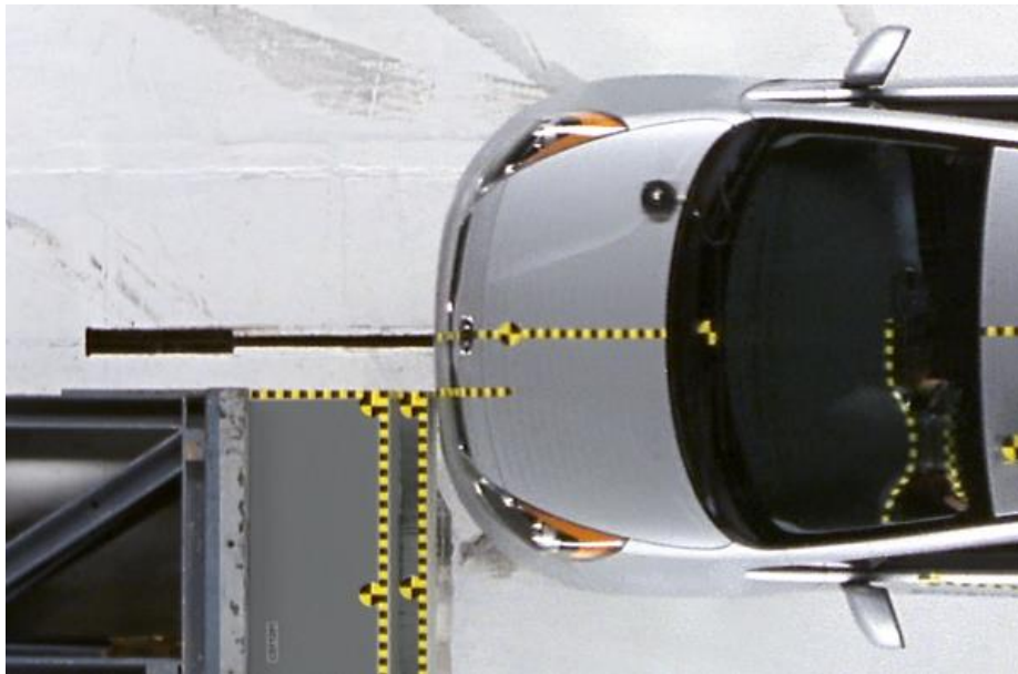
Obrázek 3.4: Náráz se 40% překrytím [4]
