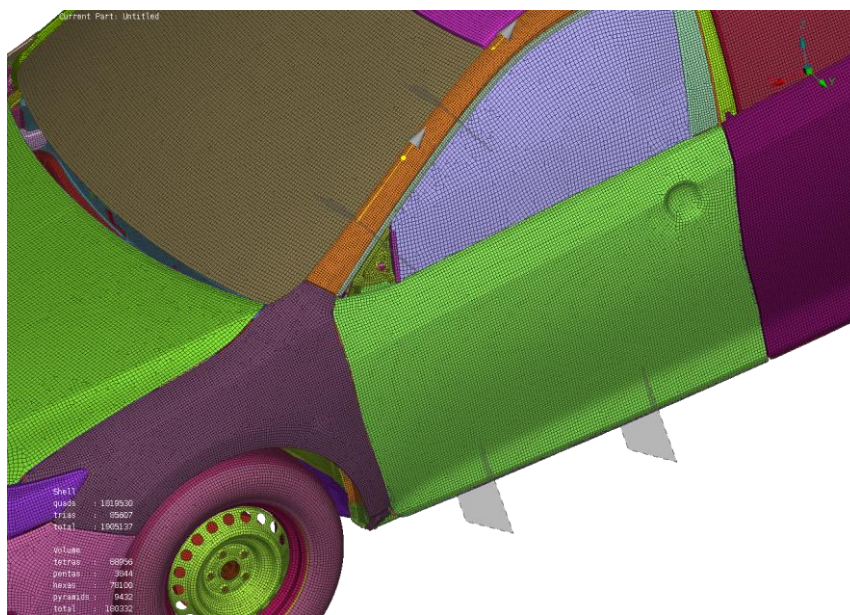
Obrázek 6.4: Section force
