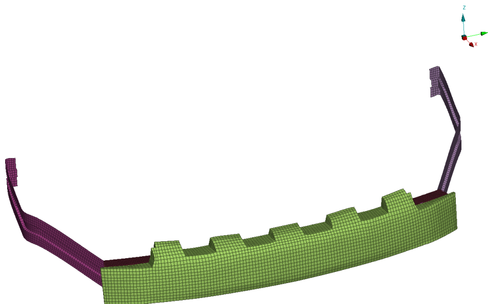
Obrázek 9.1: Přední deformační element s přidanými výztuhami
