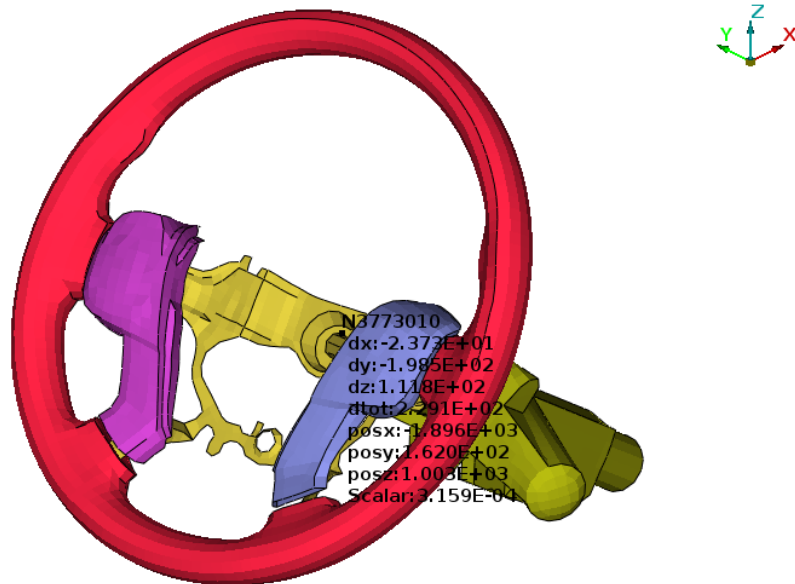
Obrázek 6.7: Posuvy koncového bodu sloupku řízení
