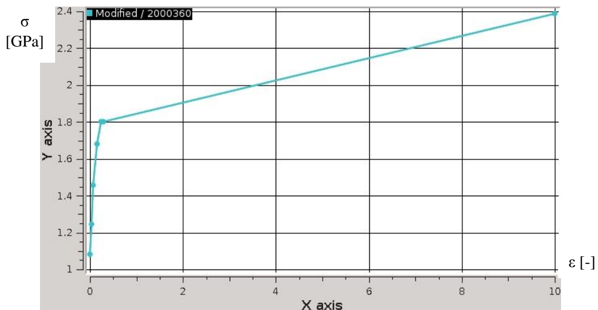
Obrázek 8.4: Závislost napětí na přetvoření nového materiálu
