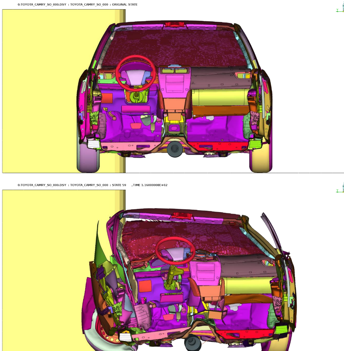
Obrázek 7.6: Srovnání interiéru před a po nárazu podle výpočtu
