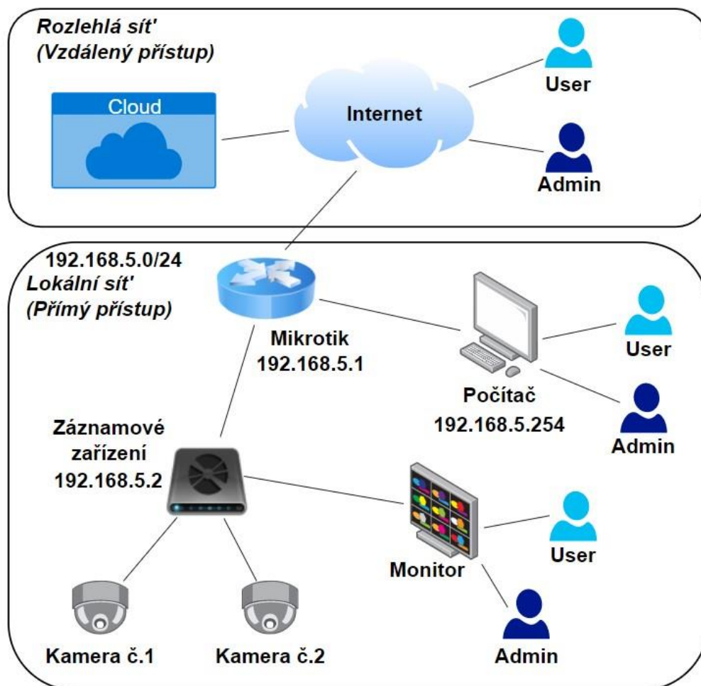
Obr. 5.2 Zapojení kamerového systému
