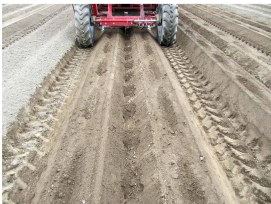
Obrázek 3: Přerušovaný žlábek na vrcholcích hrůbků a důlkování v nekolejové brázdě (Pavel Růžek)
