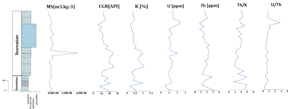
Obr.10. Profil Jesenec – křivky gama spektrometrií a magnetické susceptibility
