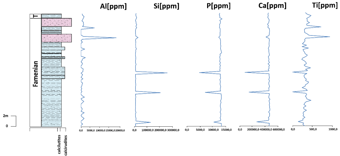
Obr.17. Grygov – křivky prvkových koncentrací Al, Si, P, Ti, Ca
