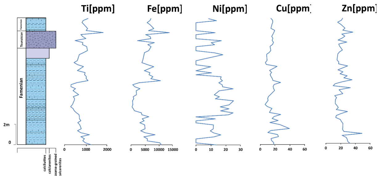
Obr. 24. Černotín – křivky prvkových koncentrací Ti, Fe, Ni, Cu, Zn
