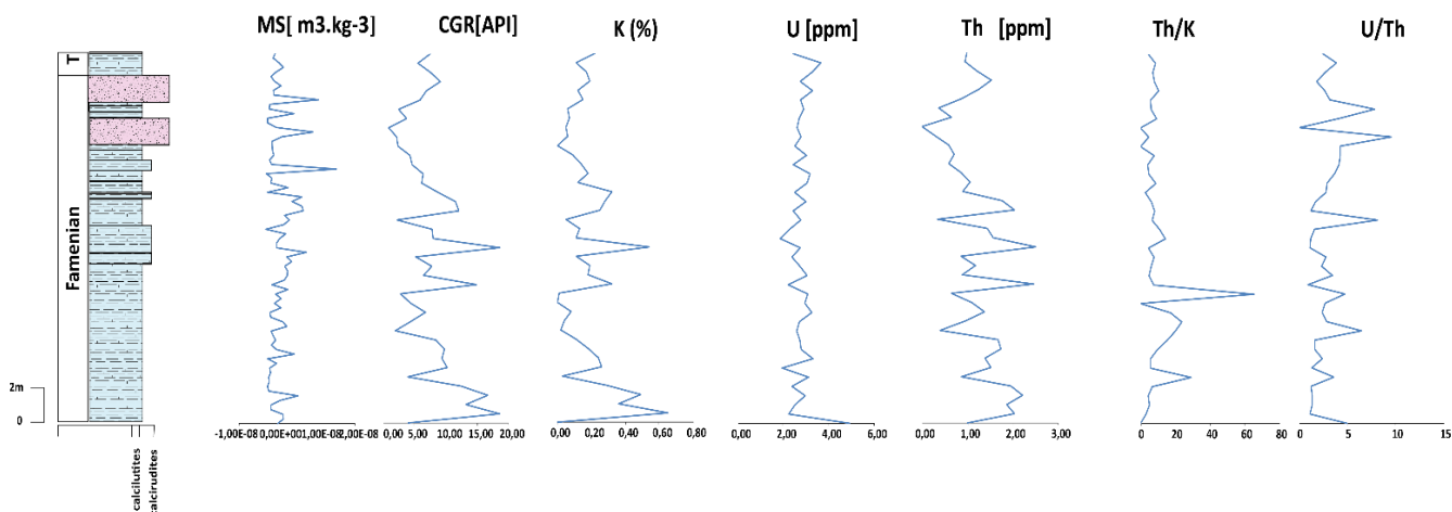
Obr.16. Grygov –měření magnetické susceptibilitě a gamaspektrometrií.
