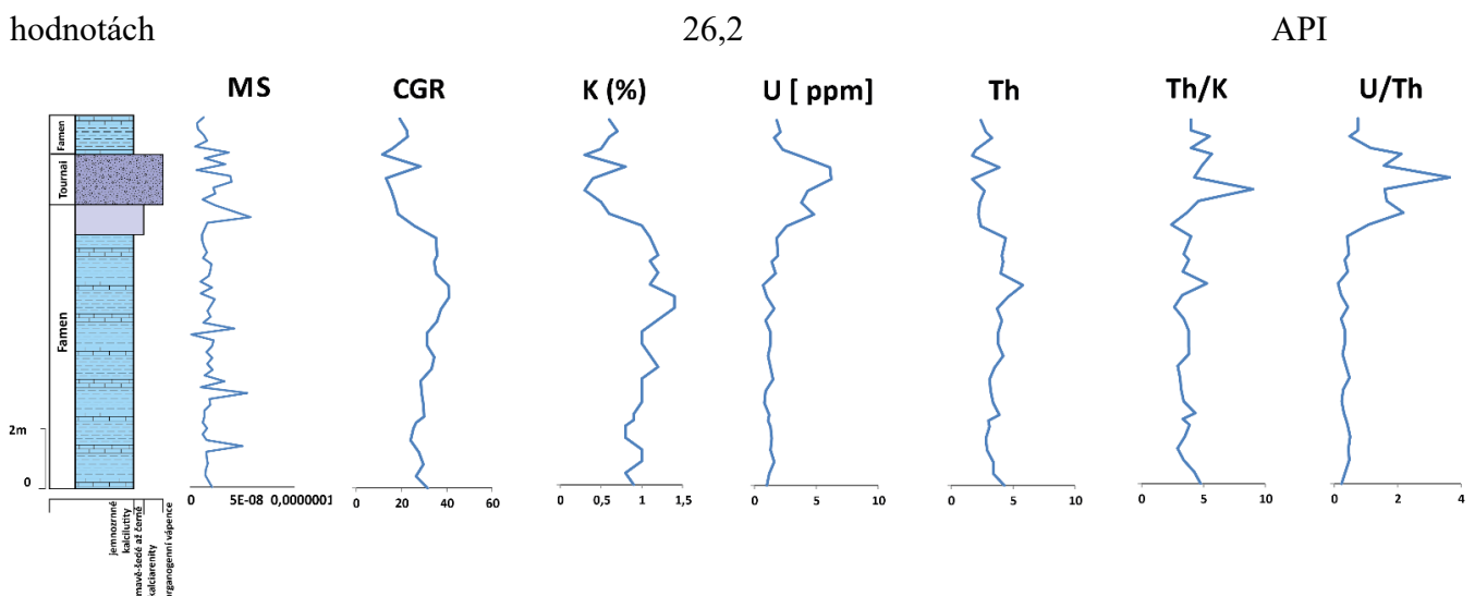
Obr.22. Černotín – křivky magnetické susceptibility a gama spektrometrií
