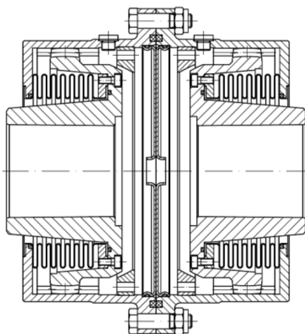
Obr 17 Zubová spojka od firmy KWD s vlnovcovým řešením[24]
