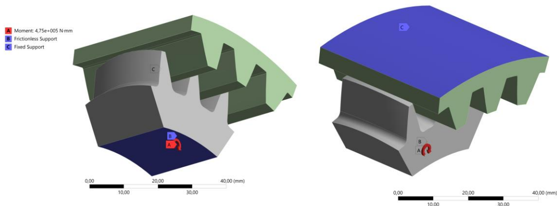
Obr. 43 Model ozubení s okrajovými podmínkami
