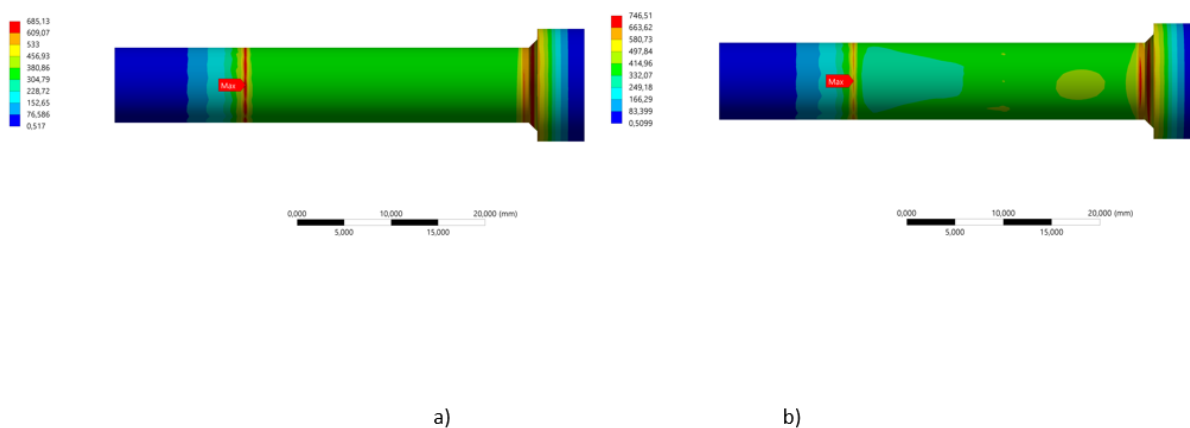
Obr. 41 Výsledky výpočtů napětí dle HMM a) první časový krok, b) druhý časový krok
