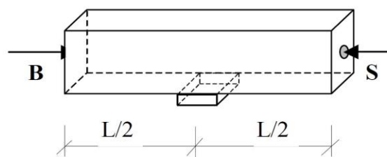
Obr. 11 Poloha snímače a budiče pro podélné kmitání [34]
