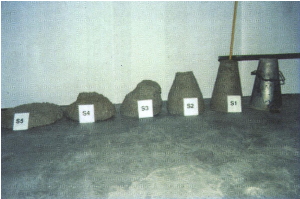
Obr. 2 Sednutí kužele betonu s různou třídou konzistence (od S5 k S1) [2]
