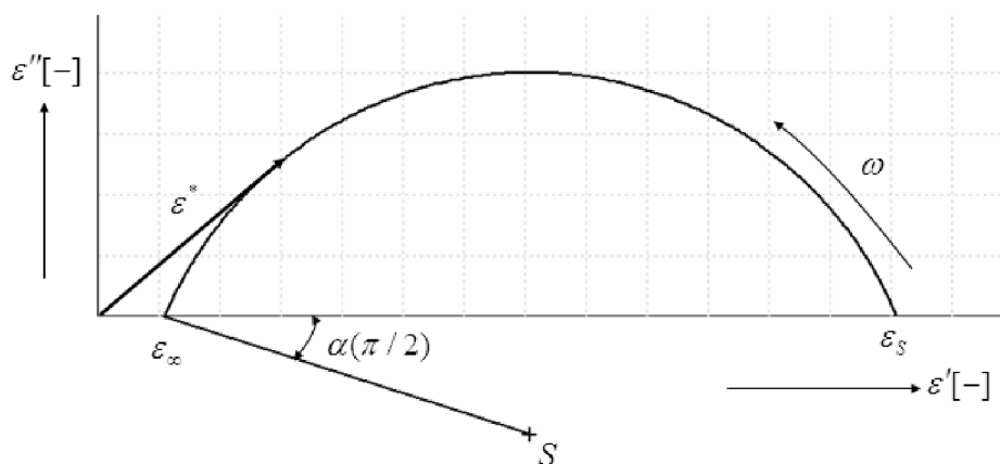
Obr. 2: Coleho-Coleho diagram
