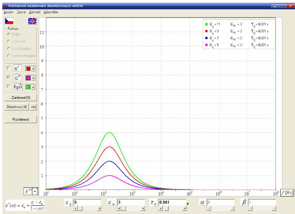
Obr. 14: Zobrazení vlivu parametru \epsilon_s na ztrátové číslo \epsilon''
