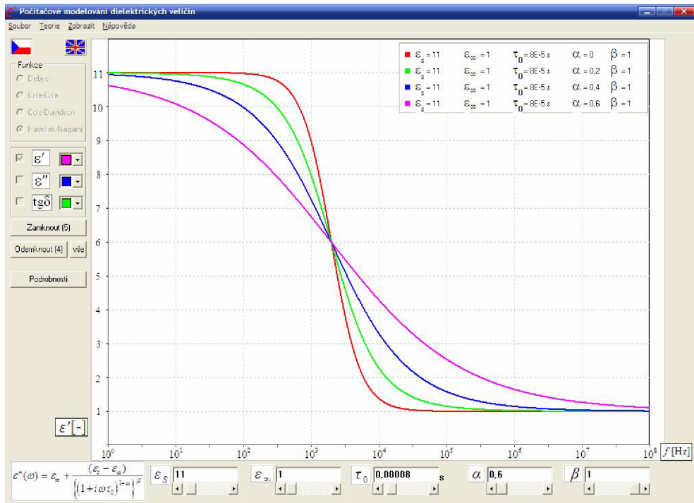
Obr. 13: Zobrazení vlivu parametru \alpha na relativní permitivitu \epsilon'
