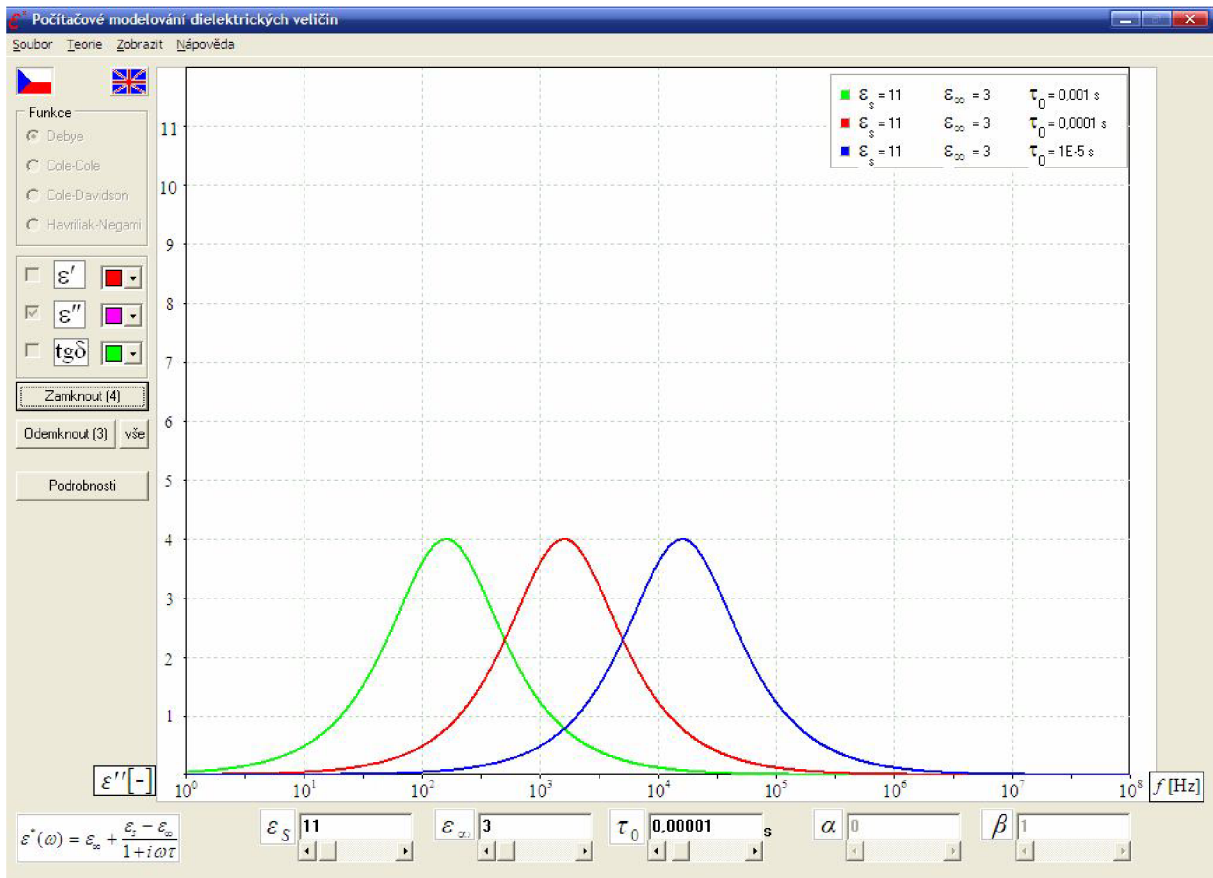
Obr. 15 : Zobrazení vlivu parametru \tau_0 na ztrátové číslo \varepsilon''
