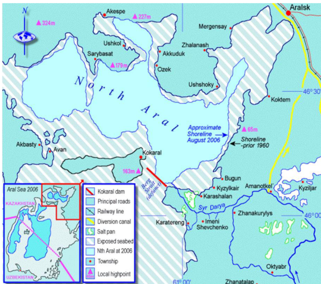
obr. 7: Projekt přehrady Kokaral. (zdroj – Oskenbayeva a kol., 2017).
