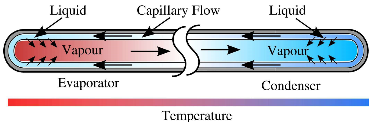
Obr. 8 Princip funkce tepelné trubice
