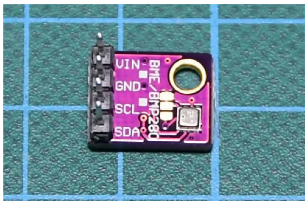
Obr. 3.5: Modul se senzorem Bosch BME280 [22].
