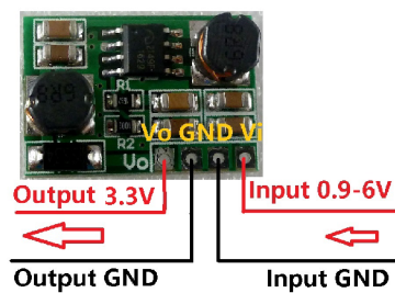
Obr. 3.10: Modul měniče buck-boost [24].
