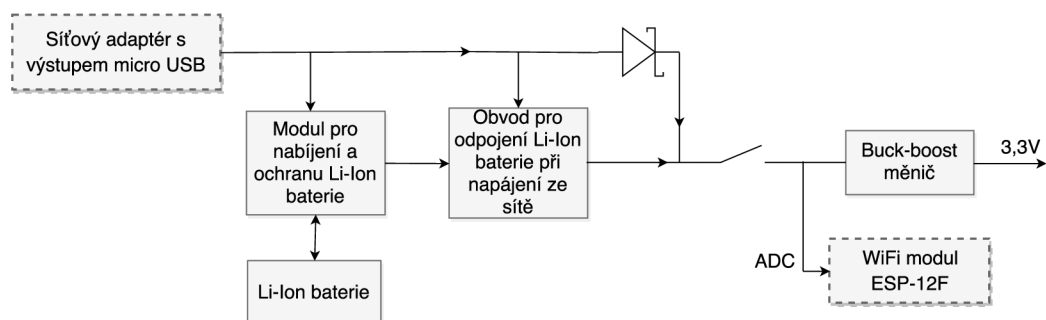
Obr. 3.7: Blokové schéma napájecího obvodu.
