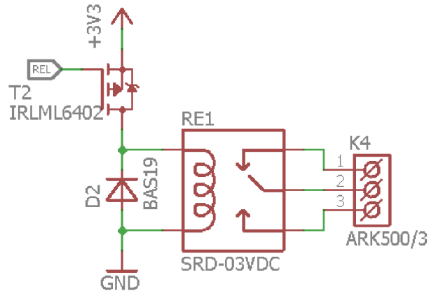
Obr. 3.6: Zapojení relé pro řízení spotřebičů.
