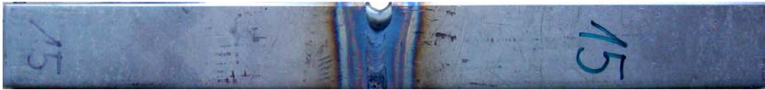
Obr. 26 Nátav vzorku č.2
