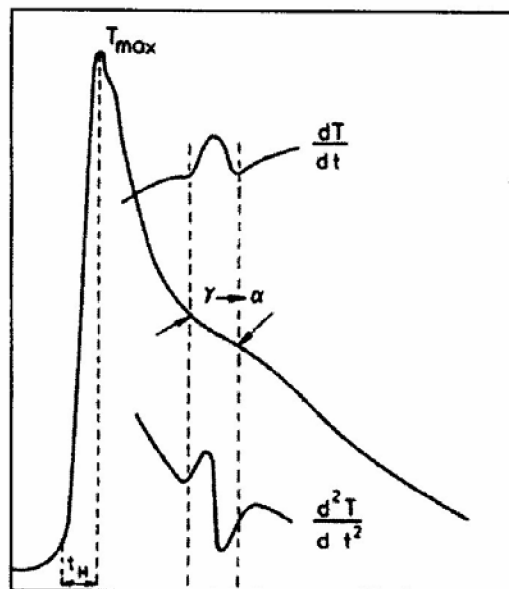
Obr. 7 Záznam teplotního cyklu pásma přehřátí s vyznačením začátku a konce přeměny \gamma \rightarrow \alpha a záznam derivate teploty podle času (1)
