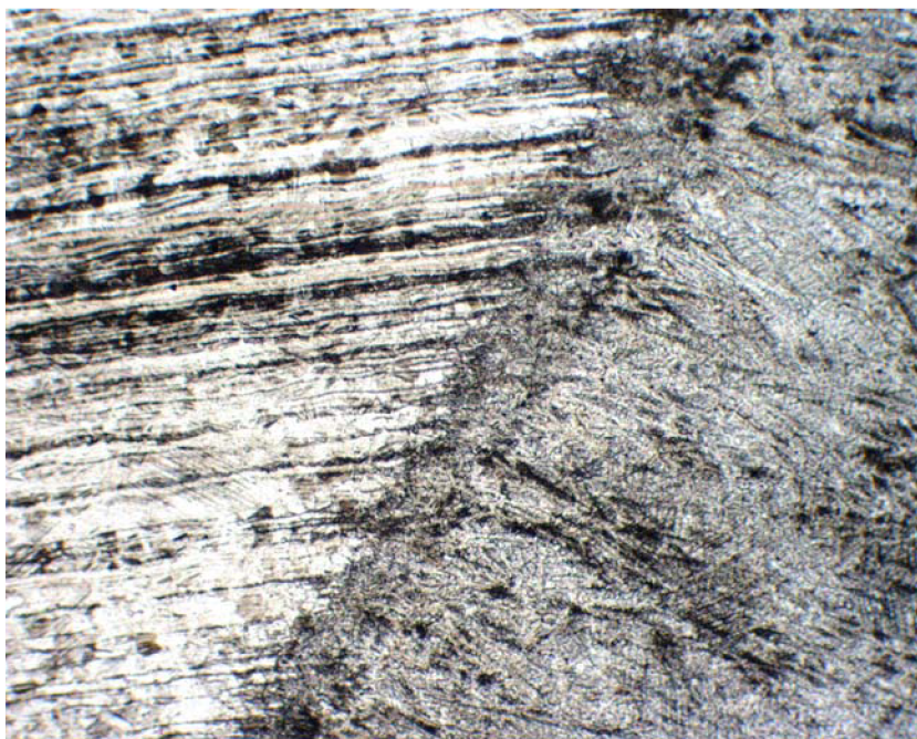
Obr. 44 Přechodová oblast
