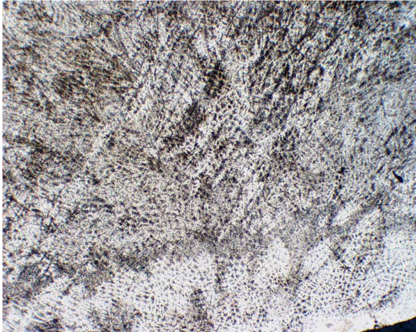
Obr. 47 Struktura nátavu
