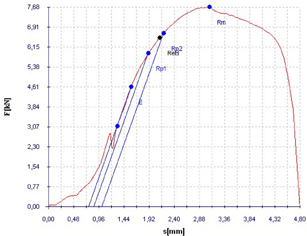
Obr. 25 Tahový diagram vzorku č.1
