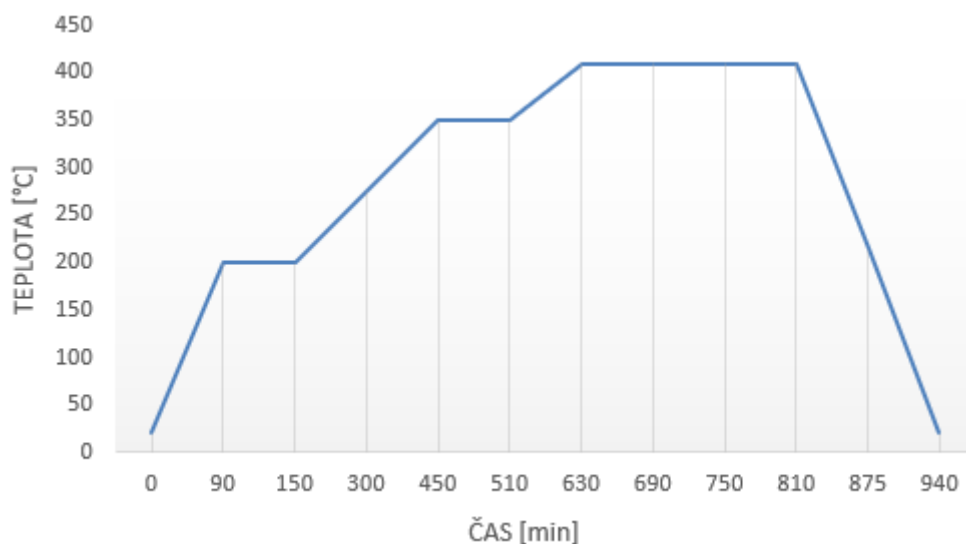
Obr. 16 Debindovací cyklus
