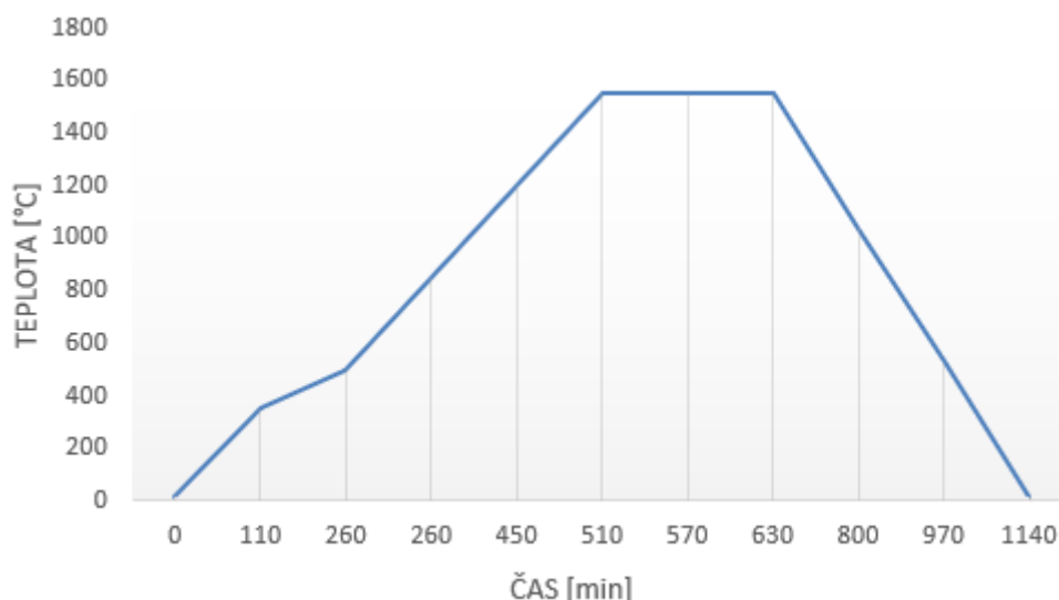
Obr. 19 Slinovací cyklus
