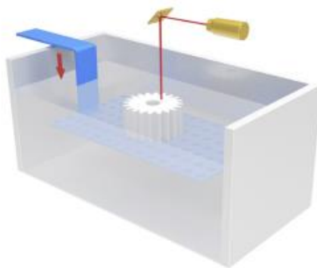
Obr. 4 Schematický diagram SLA tisku [2]
