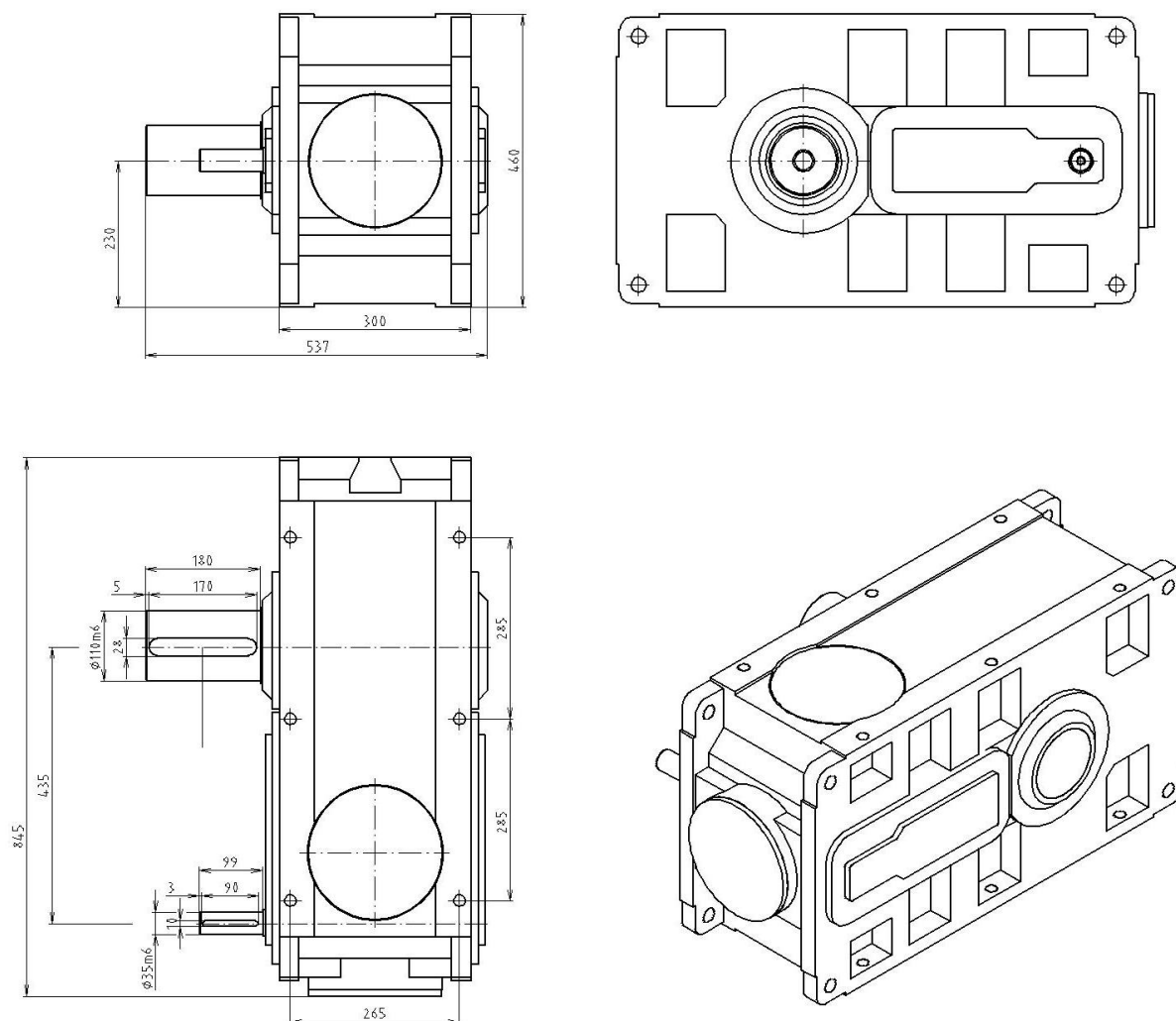
Obr. 14 Rozměry převodovky
