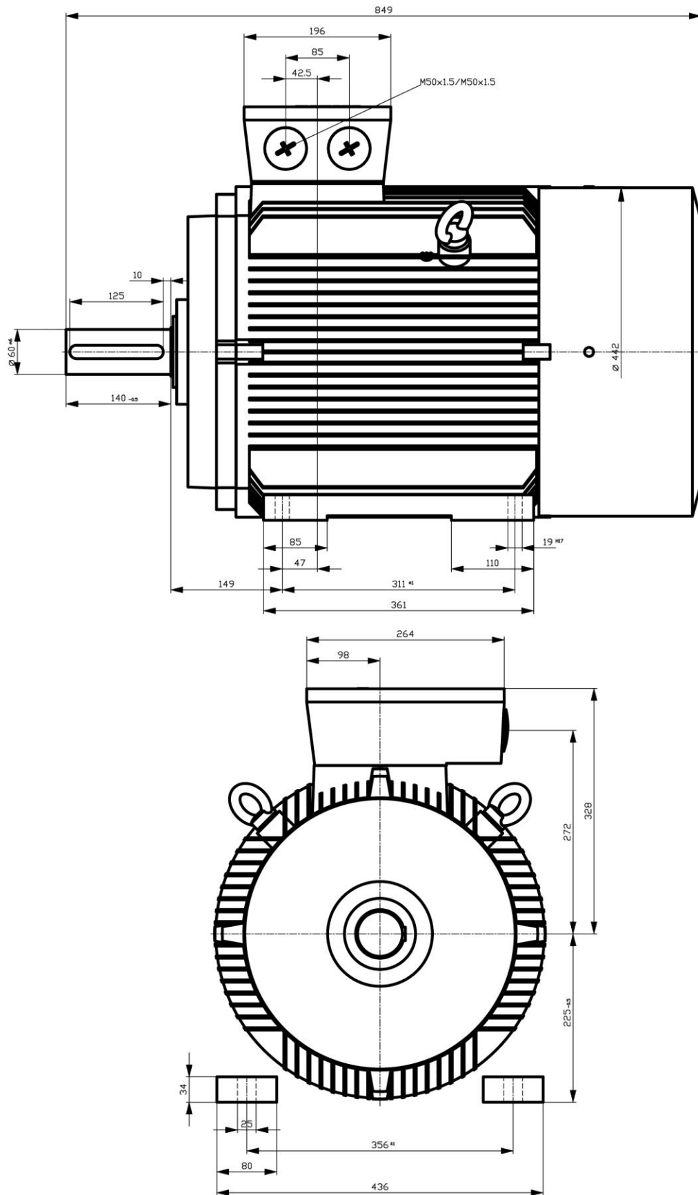
Obr. 13 Rozměry elektromotoru [13]
