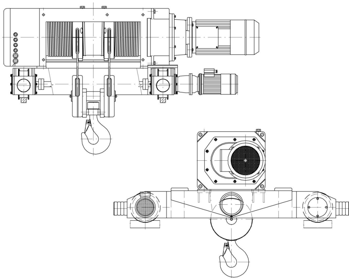
Obr. 4 Jeřábová kočka Giga řady GSM [5], str. 115
