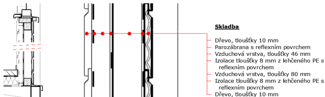
Obr. 27 Řez měřené konstrukce, včetně konstrukčního uspořádání [autor]
