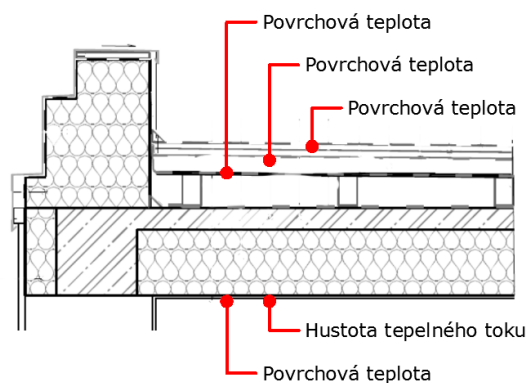
Obr. 32 Schéma rozmístění měřících čidel [autor]
