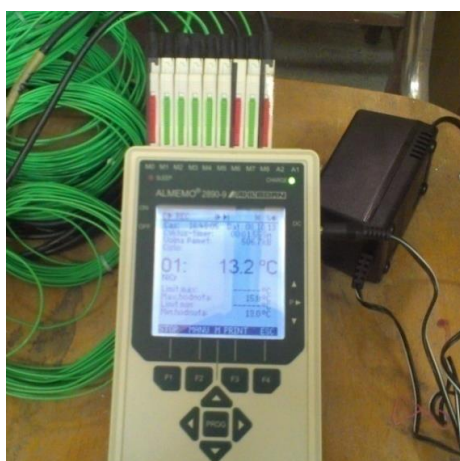
Obr. 36 Pohled na měřicí ústřednu - datalogger univerzální ALMEMO 2890-9 a osazení měřicího čidla - snímače tepelného toku a povrchové teploty [archiv autora]
