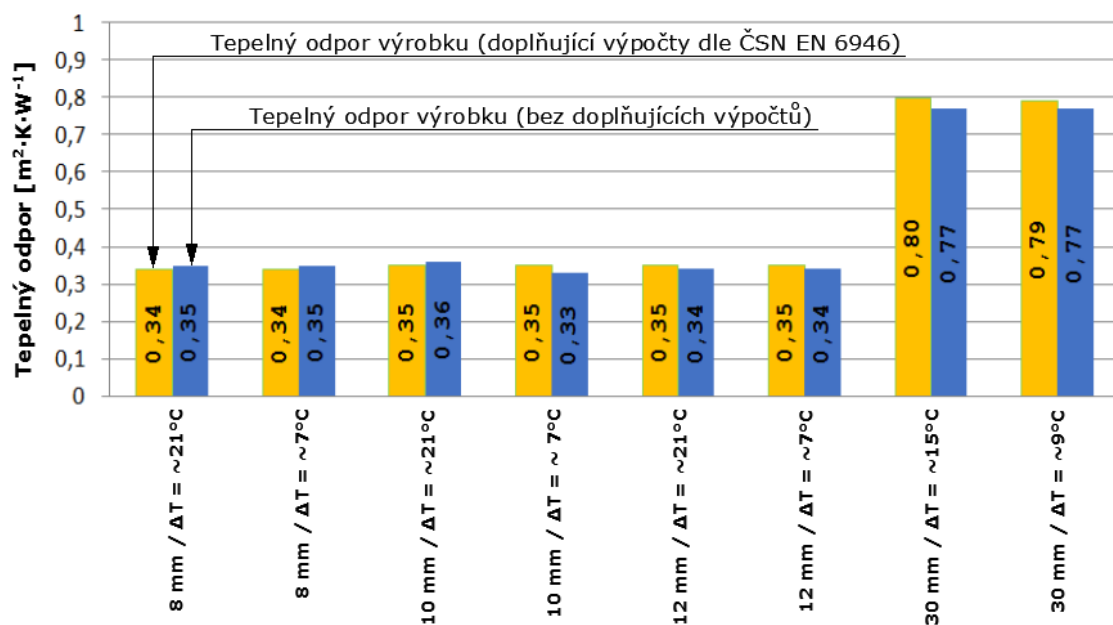
Obr. 45 Naměřené a vypočtené hodnoty tepelného odporu jádra výrobku
