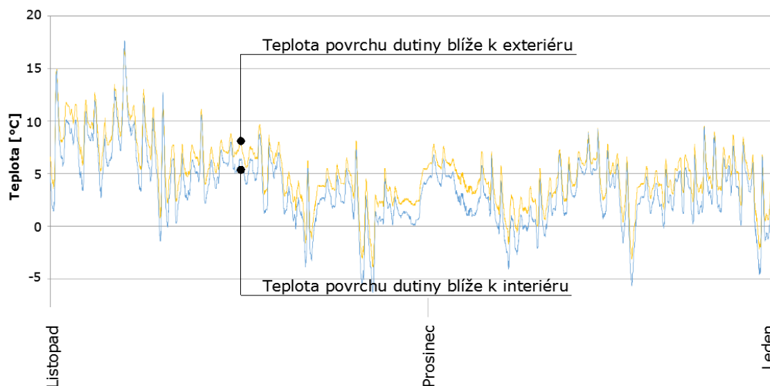
Obr. 57 Průběh měření (1. 11. 2013. – 14. 1. 2014)
