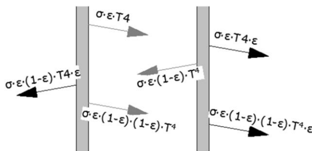
Obr. 17 Schéma výměny vyzářeného tepla mezi dvěma plochami [autor]
