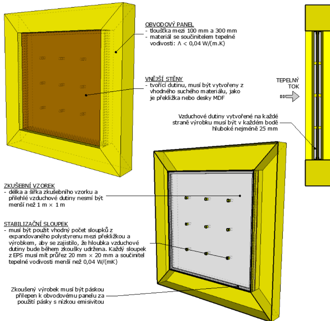
Obr. 20 Schéma typického zkušební prvku pro měření tepelného odporu izolované vzduchové dutiny metodou teplé skříně [ autor dle ČSN EN 16012]
