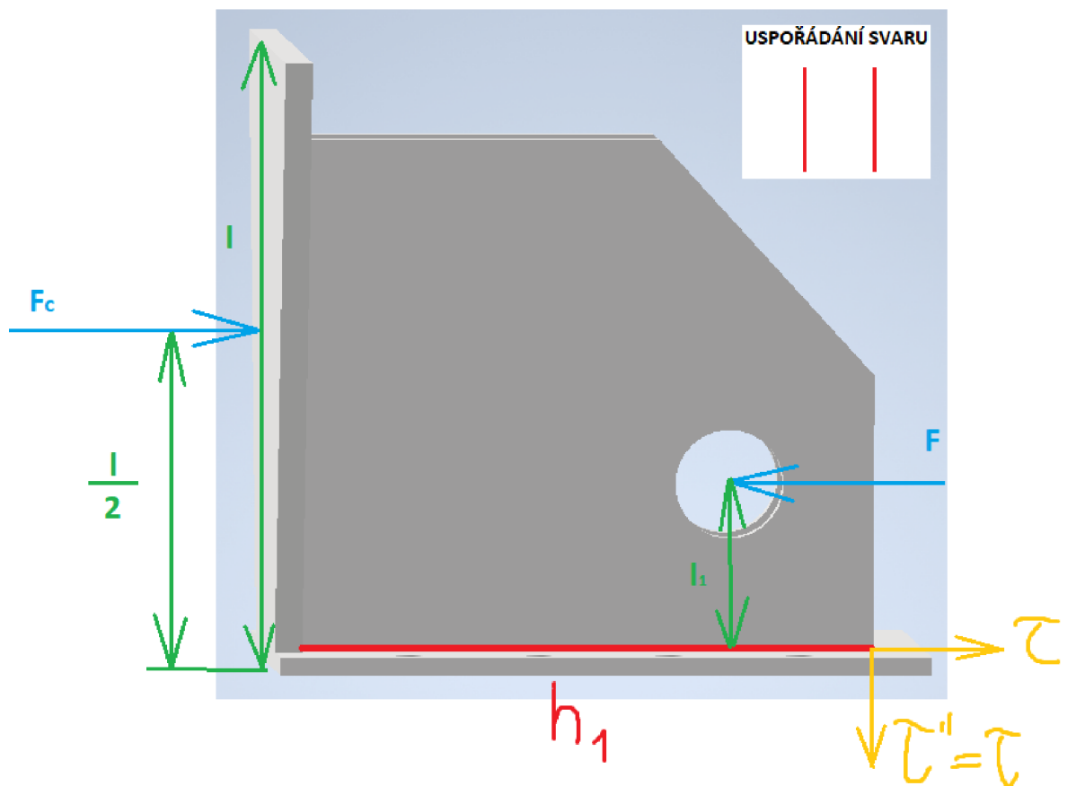
Obrázek 20 Pohyblivá konzole
