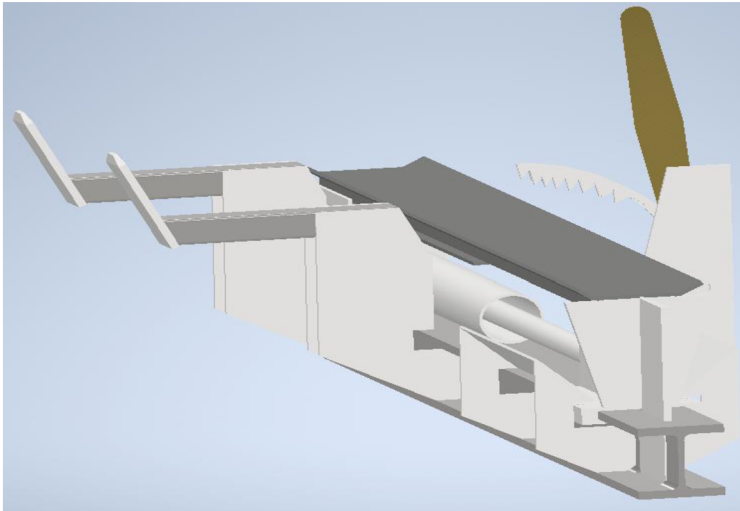
Obrázek 10 Koncepční návrh
