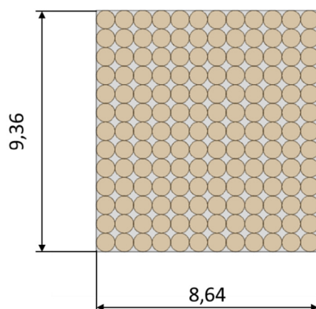
Obr. 63 Rozměry průřezu svazku vláken v milimetrech
