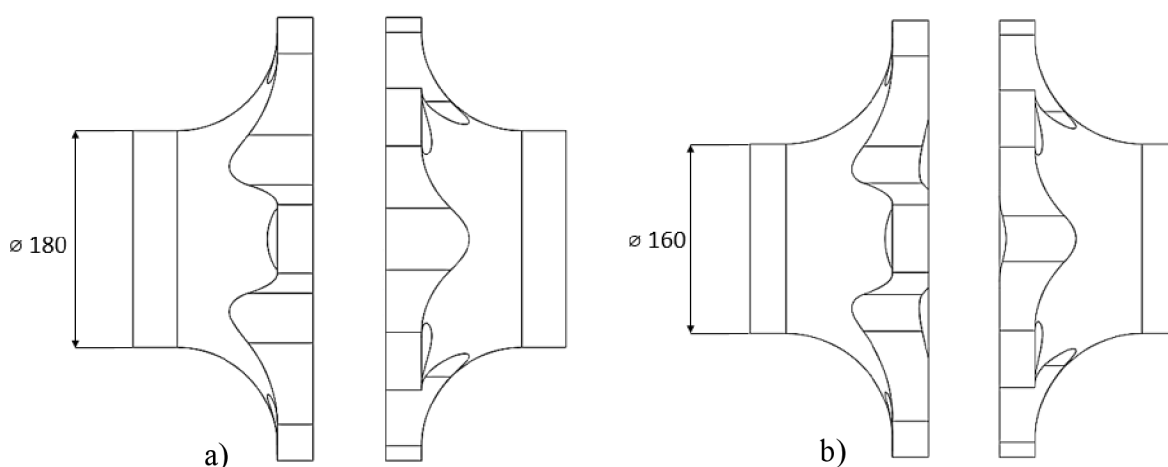
Obr. 51 Změna vnějšího průměru nábojové části vstupního un. a centrální části středového dílu. a) 1. iterace, zleva vstupní a středový díl b) 2. iterace, zleva vstupní a středový díl
