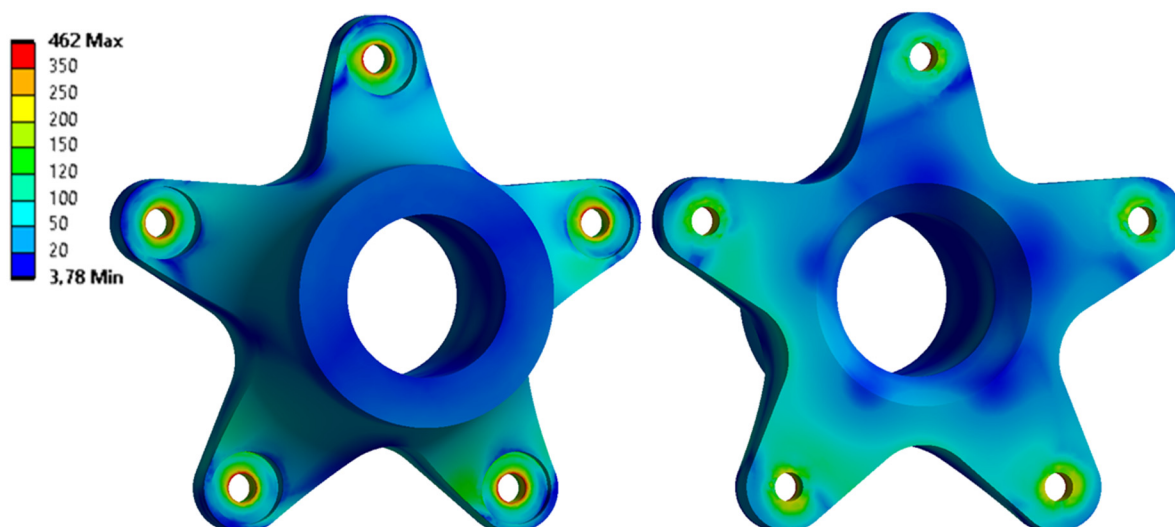
Obr. 50 Výsledné hodnoty napětí po první iteraci – středový unášče
