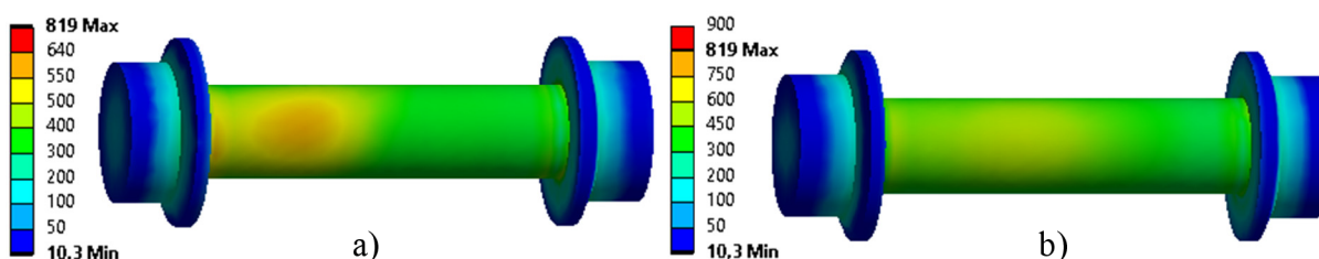
Obr. 46 Dosažené napětí na šroubech a) šrouby pevnostní třídy 8.8 b) šrouby pevnostní třídy 10.9
