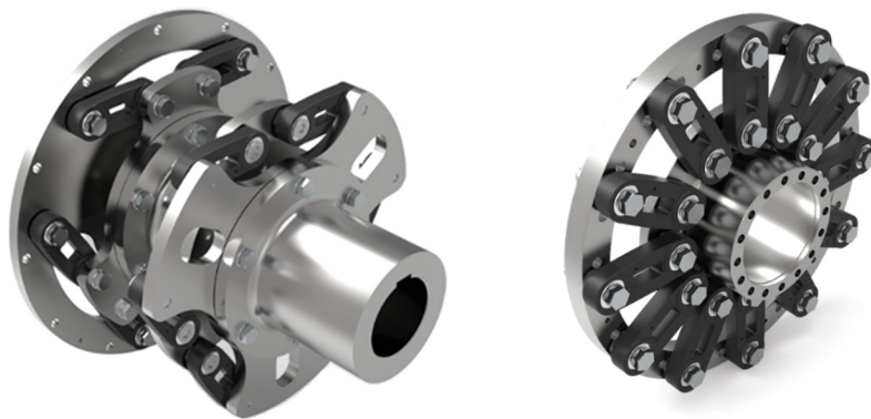
Obr. 18 Alternativní konfigurace segmentů ve spojce [33]
