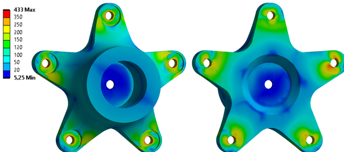
Obr. 49 Výsledné hodnoty napětí po první iteraci – vstupní unášče
