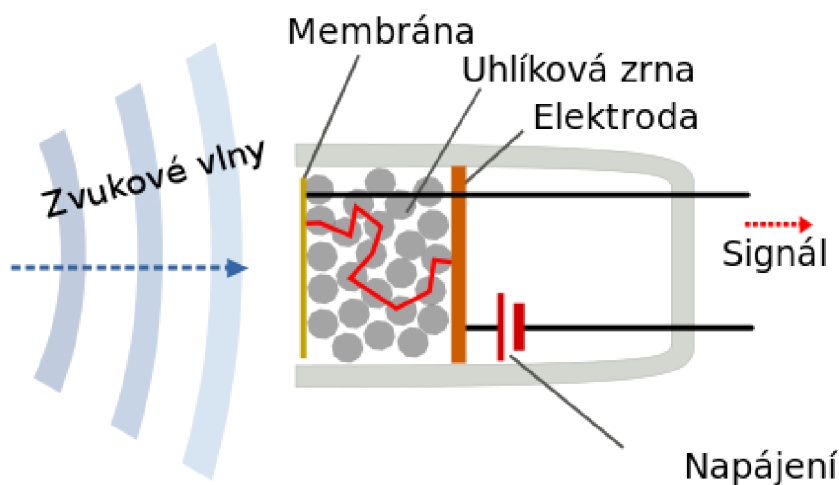
Obr. 1.6 Uhlíkový mikrofon [7]
