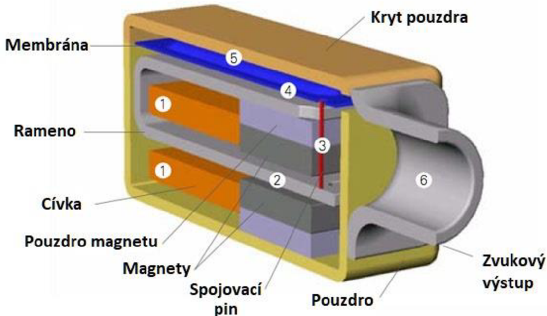
Obr. 1.2 Tlakový měnič [3]
