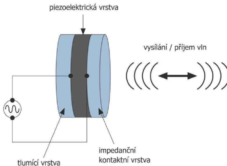
Obr. 1.5 Piezoelektrický měnič [6]
