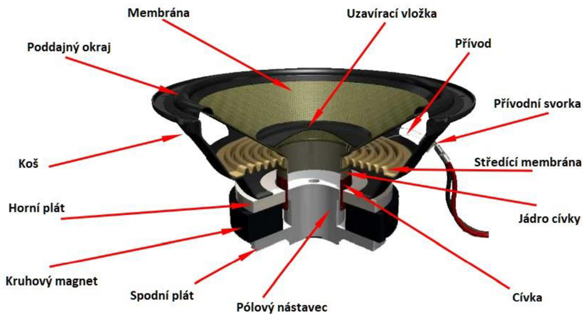
Obr. 1.1 Elektrodynamiccký měnič [2]
