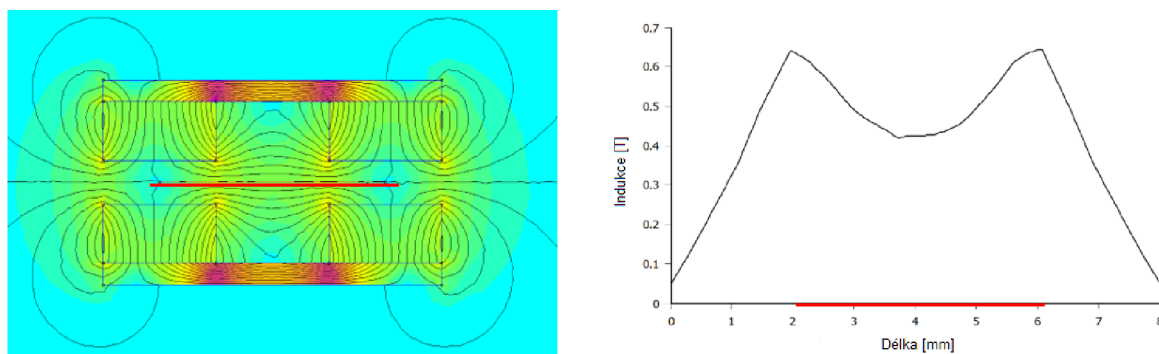
Obr. 3.6 Simulace mag. pole s grafem působení síly [18]
