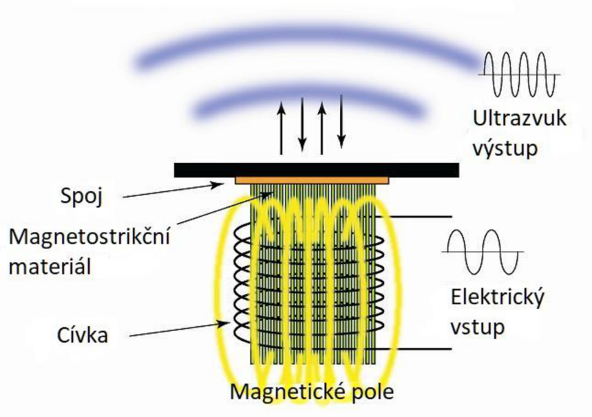
Obr. 1.4 Magnetostrikční měnič [8]
