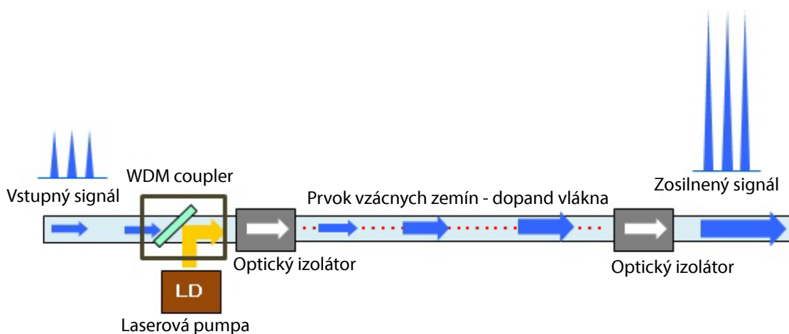
Obr. 7.1: Schéma optického zosilňovača dopovaného prvkami vzácnych zemín [9].
