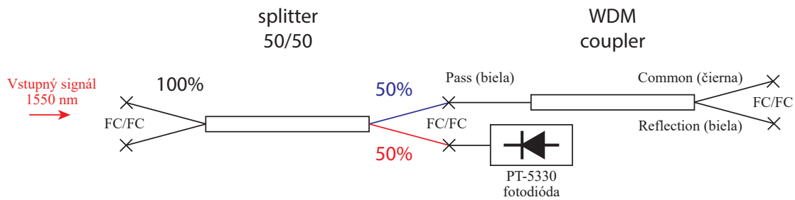
Obr. 4.13: Schéma zapojenia 50/50 splittra č. 1.
