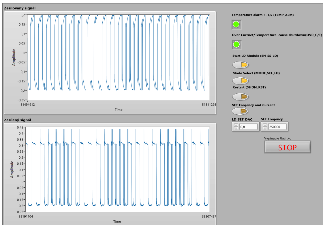
Obr. 5.5: Ovládací panel
