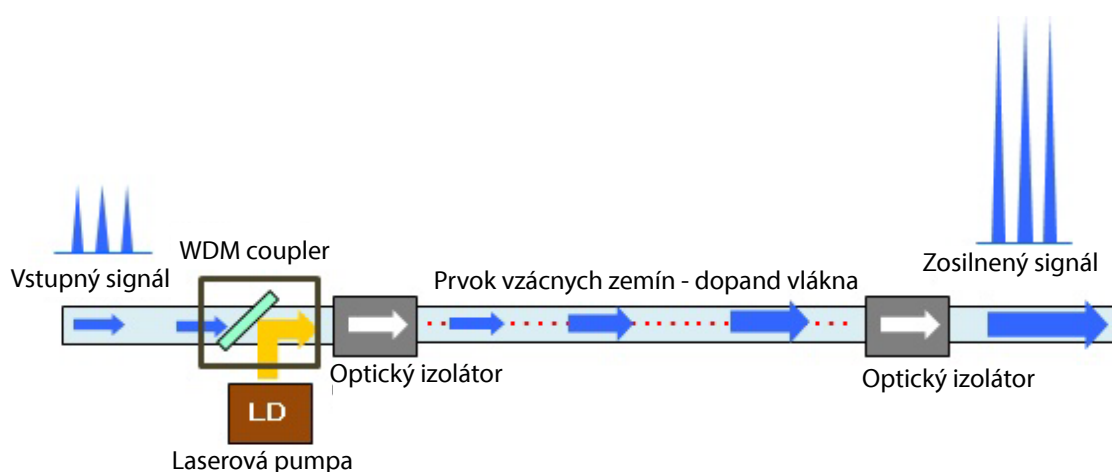
Obr. 3.2: Schéma optického zosilňovača dopovaného prvkami vzácnych zemín [9].
