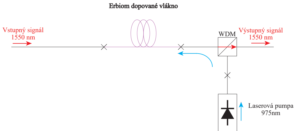
Obr. 7.4: Schéma spätného čerpania
