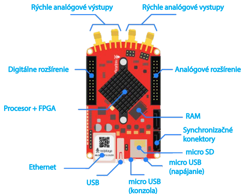
Obr. 4.2: Schéma zariadenia Red Pitaya 125-14 [12].
