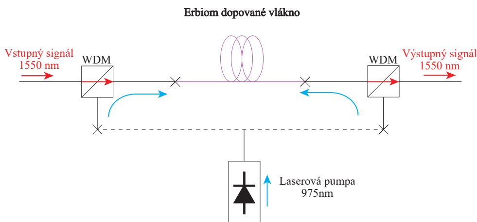
Obr. 4.9: Schéma obojstranného čerpania
