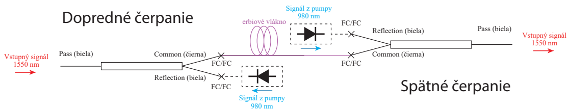
Obr. 4.12: Schéma zapojenia WDM couplerov
