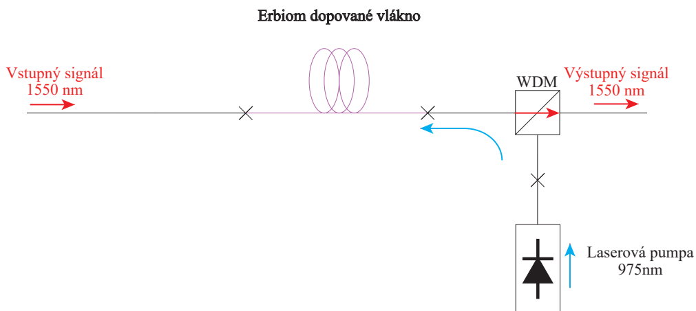
Obr. 4.8: Schéma spätného čerpania
