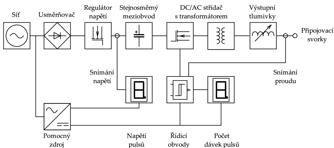
Obr. 3.2: Blokové schéma vysokonapětového generátoru.
