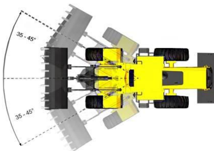
Obr.5 Řízení děleným kloubovým rámem[23]
