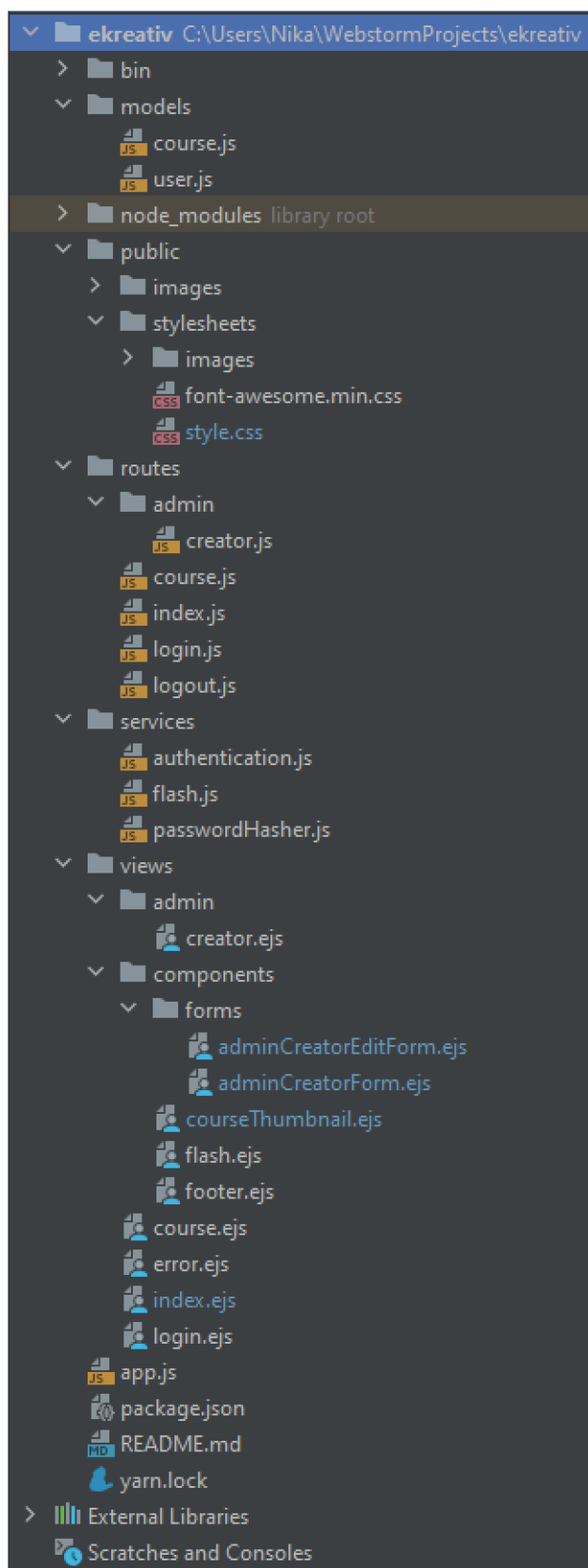
Obrázek 14 Struktura kódu e-kreativ
