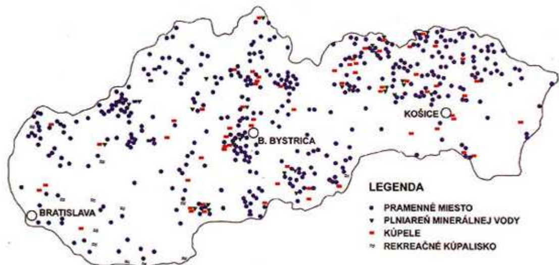
Obr. 1 – Rozložení minerálních a termálních pramenů na území Slovenska (zdroj: www.sazps.sk )
