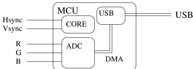
Obrázek 5.2: Blokové schéma architektury VGA grabberu využívající MCU s vestavěným ADC převodníkem
