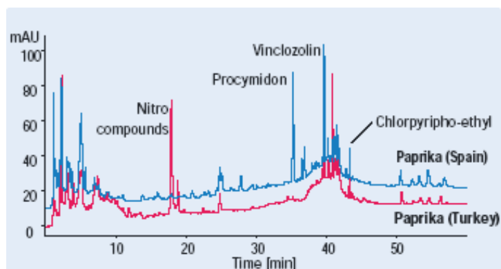
Obrázek 10: Chromatogram - (převzato: Schulzová 2006)
