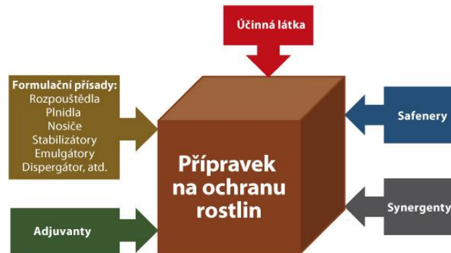
Obrázek 2: Základních složky obsažené v přípravku na ochranu rostlin (převzato: Prokop 2017)
