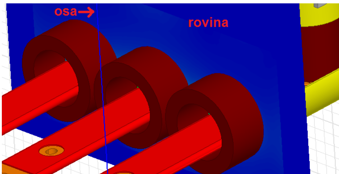
Obr. 6-2 Umístění roviny (modrá osa nesouvisí s modelem)
