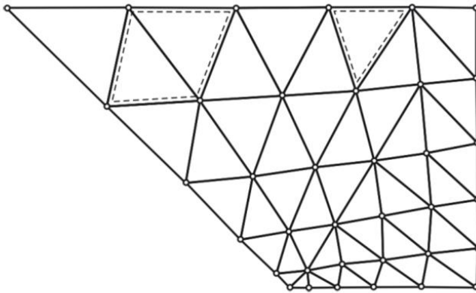
Obr. 3-1 Síť konečných prvků a jejich uzly (1 str. 30)
