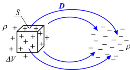
Obr. 2-1 Příklad zřídlového pole (1 str. 10)
