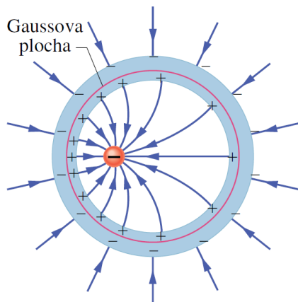
Obr. 2-5 Nehomogenně rozložený náboj uvnitř vodivé koule (3 str. 626)
