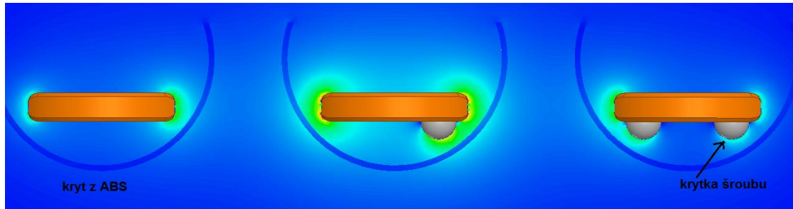
Obr. 7-6 Rozložení VIEP šroubů s krytkami, škála viz Obr. 7-8
