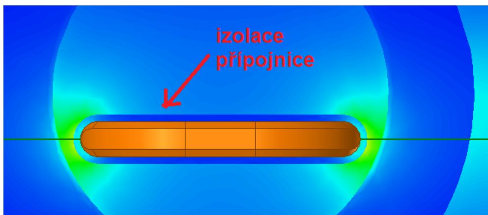
Obr. 6-4 Detail rozložení VIEP okolo prostřední přípojnice škála viz Obr. 6-1 (zelená přímka je osa!)
