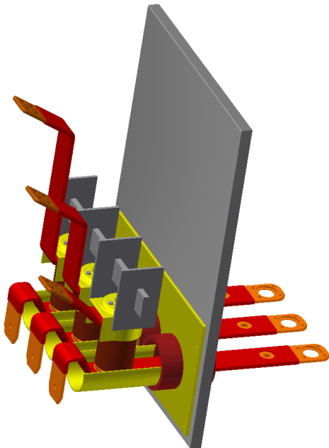
Obr. 5-2 Zjednodušený model – odstraněný systém přípojníc B
