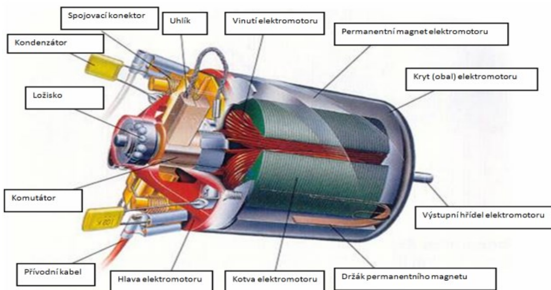
Obrázek 4 elektromotor [10]
