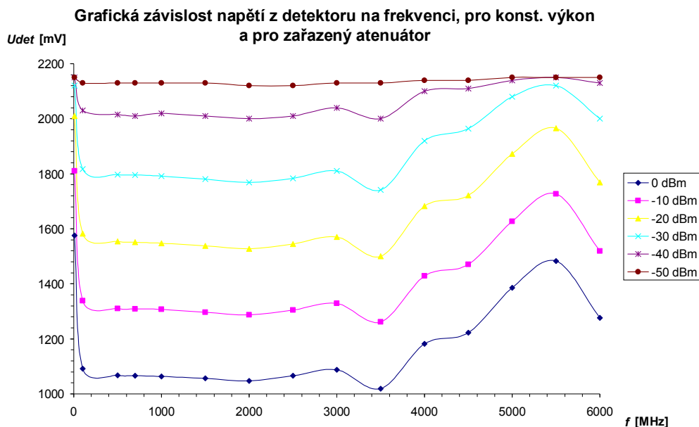
Obrázek 65. Grafická závislost napětí U_{det} na frekvenci pro zvolené hodnoty výkonů, se zařazeným atenuátorem ochrany vstupu
