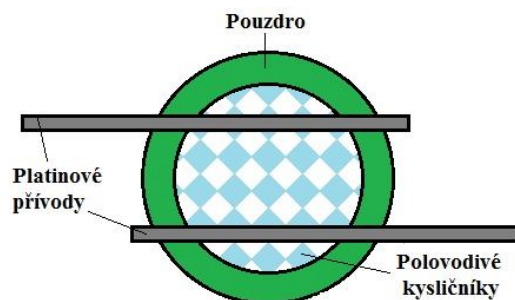
Obrázek 12. Konstrukce termistorů
