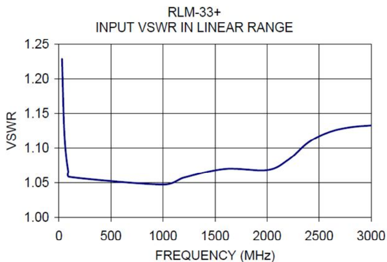
Obrázek 49. Výstupní poměr VSWR limiteru RLM-33+ [16]
