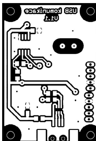
Rozměr desky 41,9 x 60,9 [mm], měřítko M1:1
