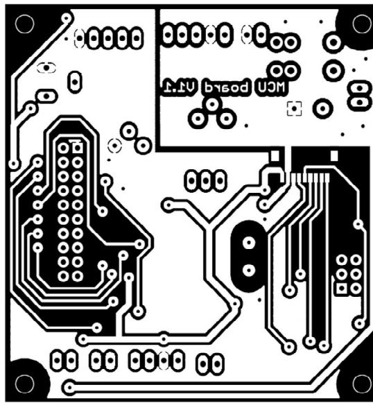
Rozměr desky 78,0 x 72,88 [mm], měřítko M1:1
