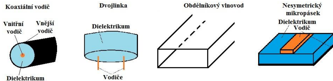
Obrázek 6. Vlnovodné struktury
