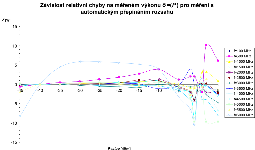
Obrázek 90. Grafická závislost relativní chyby výpočtu na měřeném výkonu
