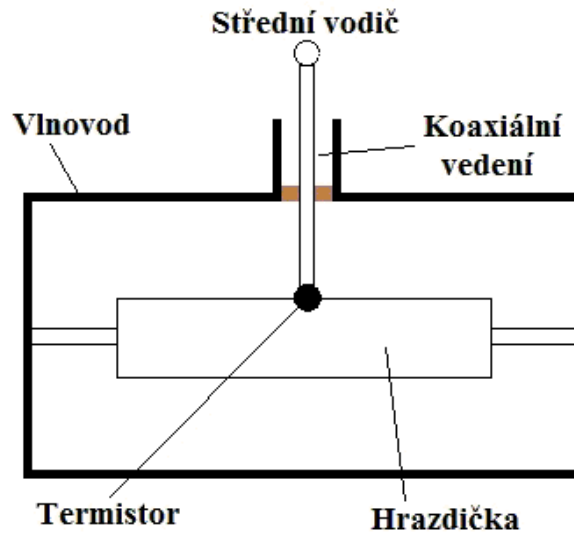
Obrázek 14. Konstrukční provedení termistorové měřící hlavice
