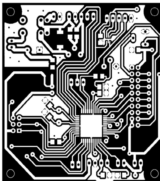
Rozměr desky 78,0 x 72,88 [mm], měřítko M1:1
