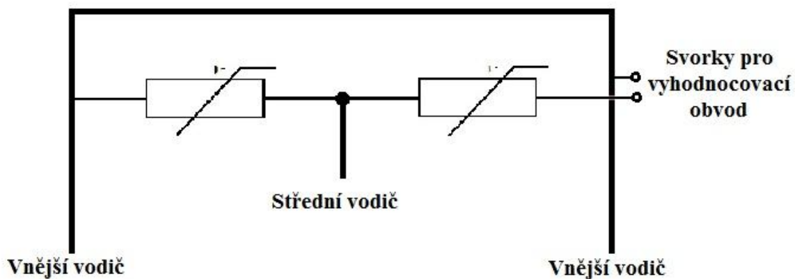
Obrázek 13. Konstruktivní provedení koaxiální termistorové měřící hlavice
