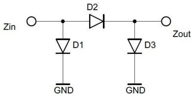
Obrázek 45. Aktivní útlumový článek PI
