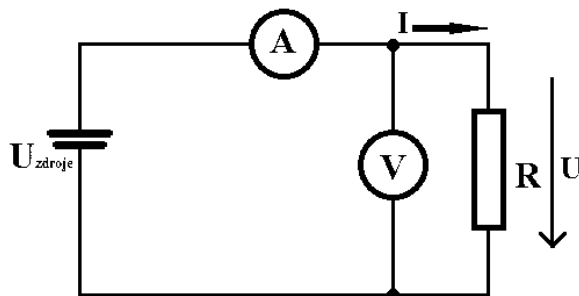
Obrázek 7. Schéma zapojení pro měření výkonu
