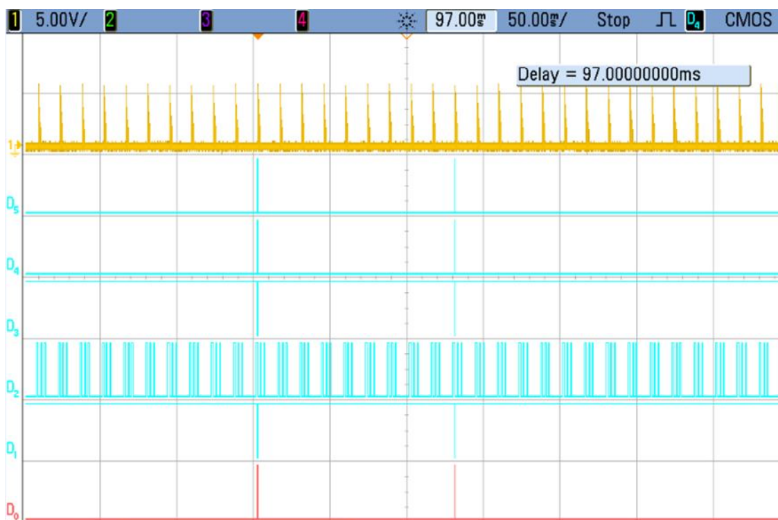
Obrázek 82. Změřené časové průběhy SPI komunikace pomocí logického analyzátoru při stisku klávesy, D0-CHANGE, D1-SS neg., D2-SCK, D3-SS neg., D4-MOSI, D5-MISO, 1-shluk měřících burstů.
