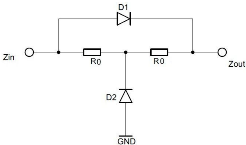
Obrázek 46. Aktivní útlumový článek T
