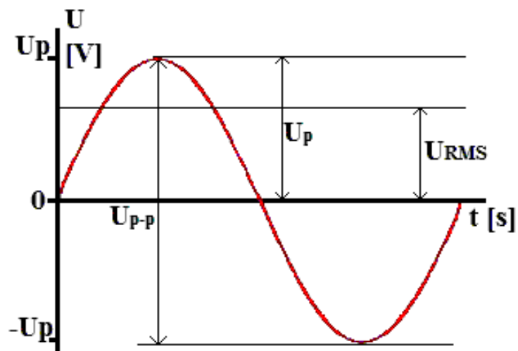
Obrázek 8. Okótovaný sinusový průběh signálu
