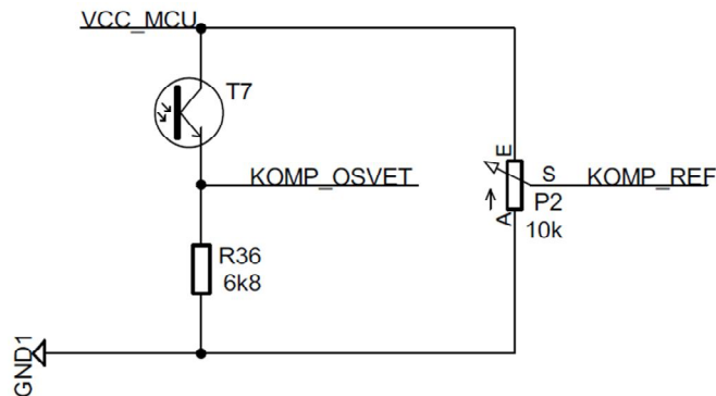
Obrázek 69. Schéma zapojení snímače osvětlení
