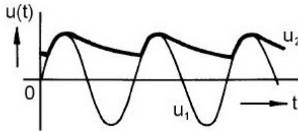
Obrázek 22. Průběh napětí na vstupu a výstupu diodového detektoru [4]
