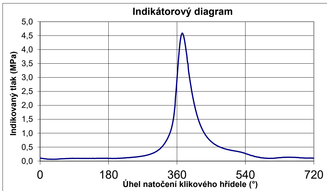
Obr. 2 Indikátorový diagram.
