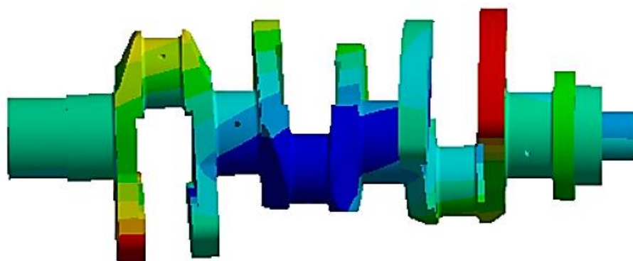
Obr. 39 10. vlastní tvar, frekvence 570,2 Hz.
