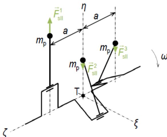
Obr. 13 Setrvačné síly posuvných částí II. řádu [2].
