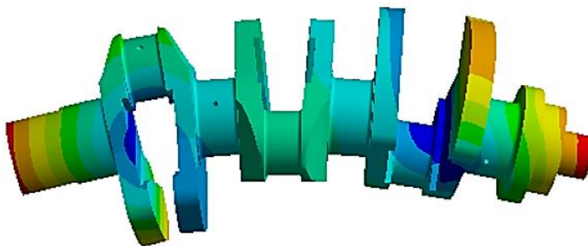
Obr. 37 8. vlastní tvar, frekvence 283,1 Hz.
