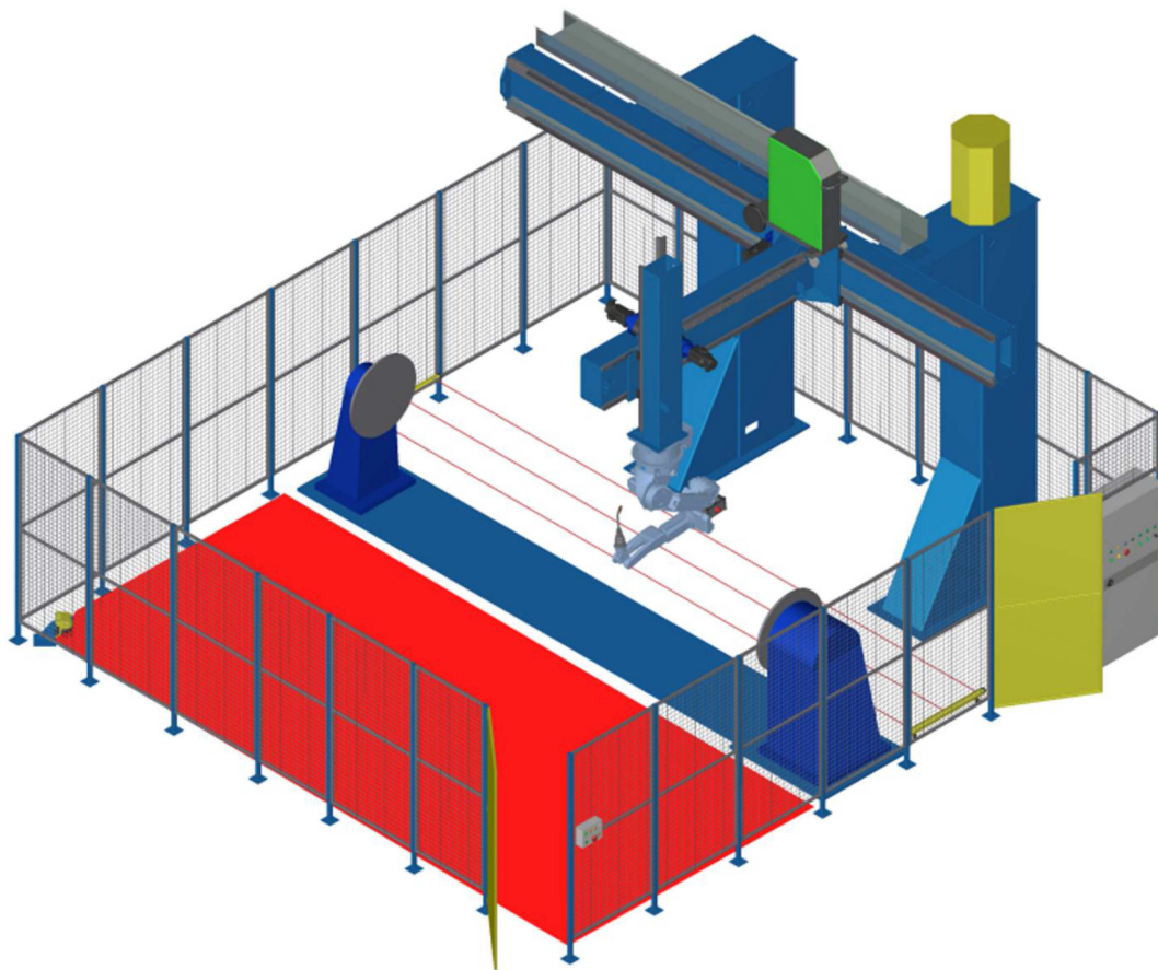
Obr. 35) Robotizované pracoviště s robotem zavěšeným na portálu nad jednoosým horizontálním polohovadlem [12]
