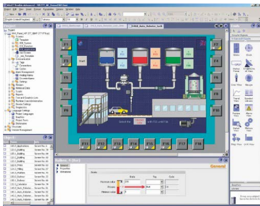
Obrázek 7: WinCC flexible [13]
