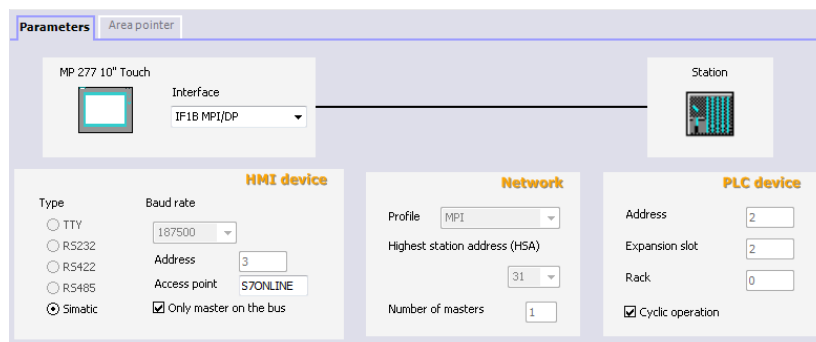
Obrázek 11: Nastavení komunikace
