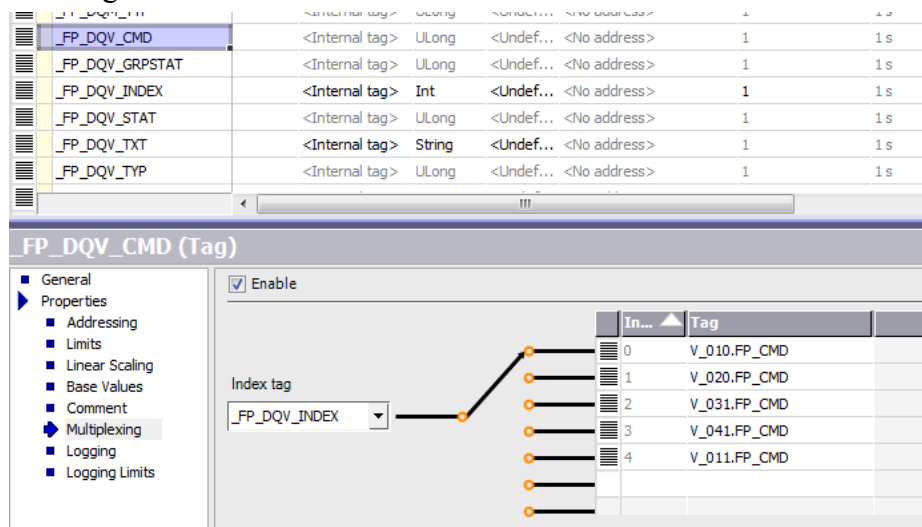
Obrázek 35: Funkce Multiplexing
