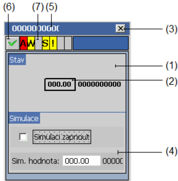
Obrázek 31: FACEPLATE okna s detaily pro analogový vstup
