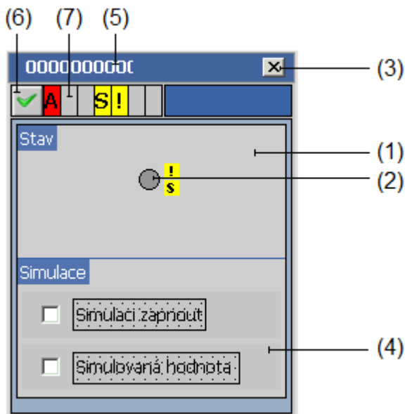
Obrázek 29: FACEPLATE okna s detaily pro digitální vstup
