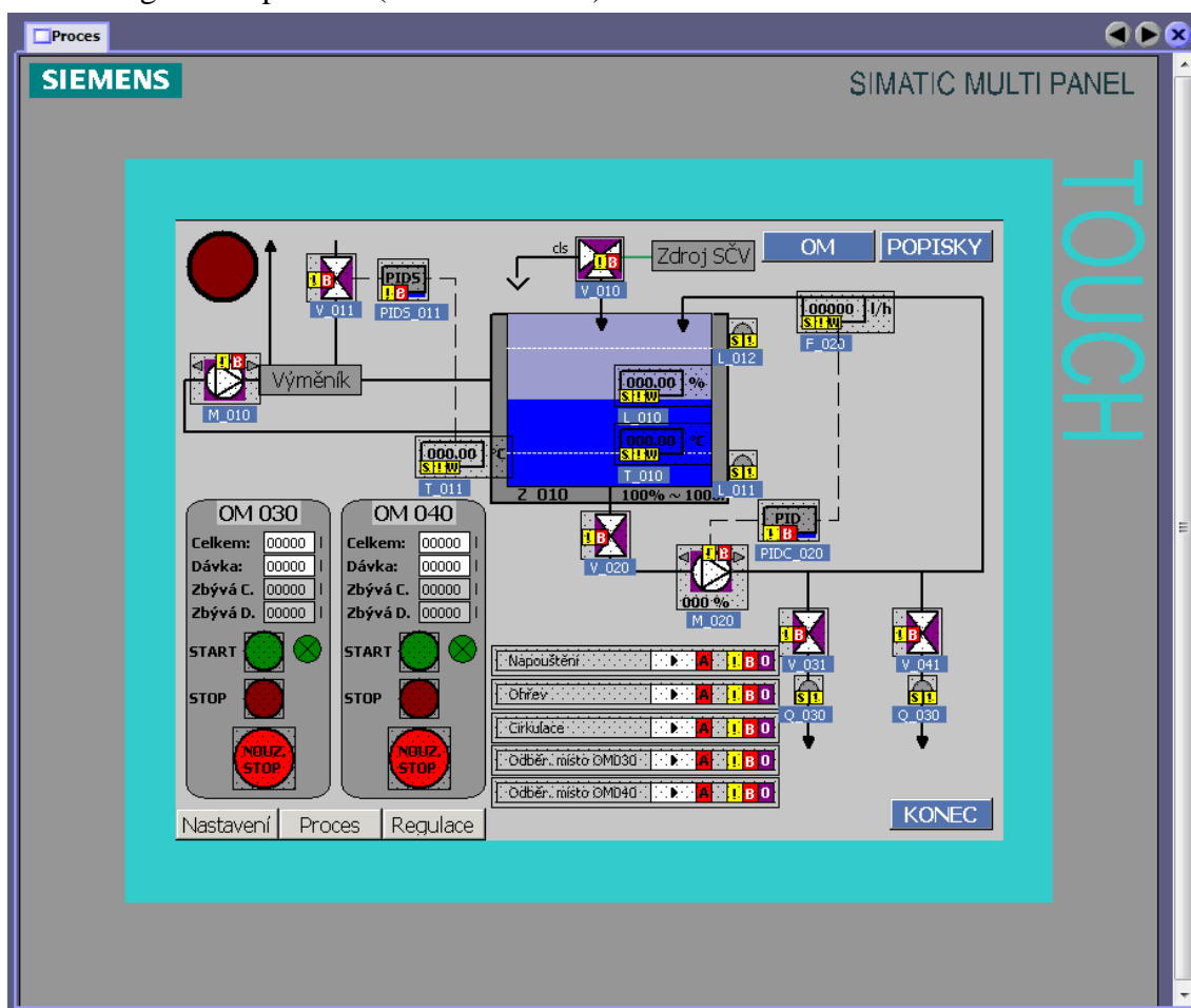
Obrázek 49: Obrazovka procesu
