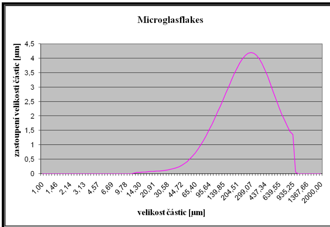
Graf 4.1 Graf velikosti částic - referenční plnivo.
