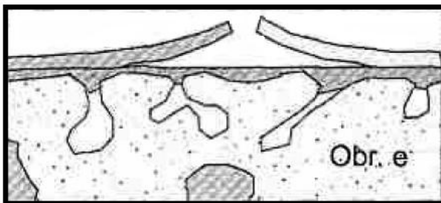
Obr. 2.6 porušení soudržnosti mezi vrstvami
