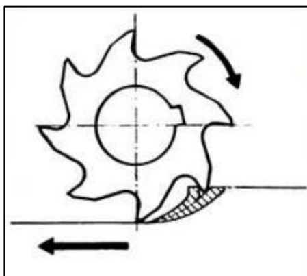
Obrázek 3: Sousedné frézování [2]
