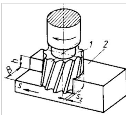
Obrázek 1: Čelní frézován [2]
