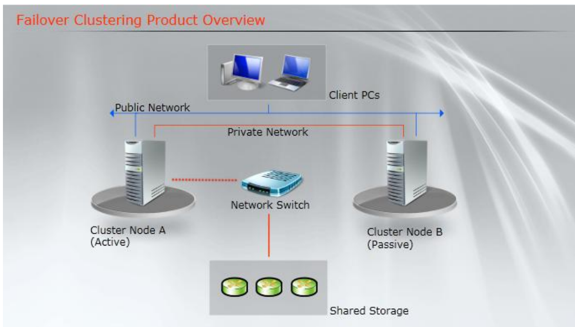
Obrázek 5: Cluster
