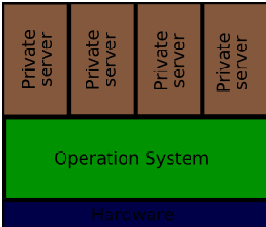
Obrázek 1: Schéma OS-virtualizace
