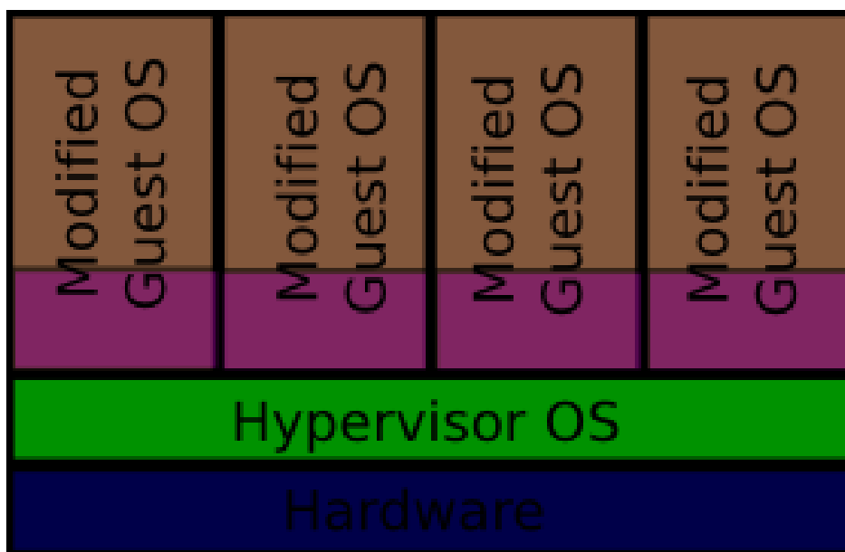
Obrázek 3: Schéma paravirtualizace
