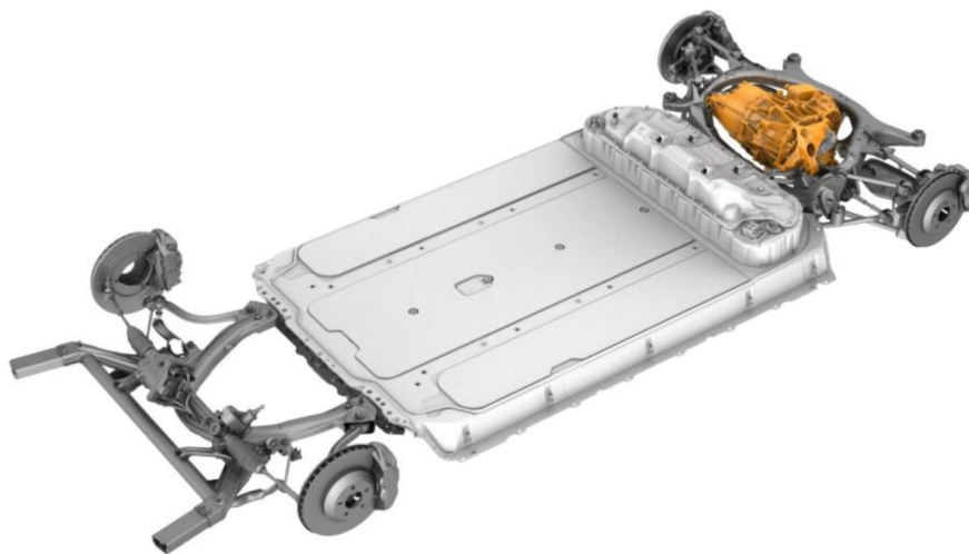
Obrázek 9 Povozeček EV s elektromotorem na zadní nápravě [32]
