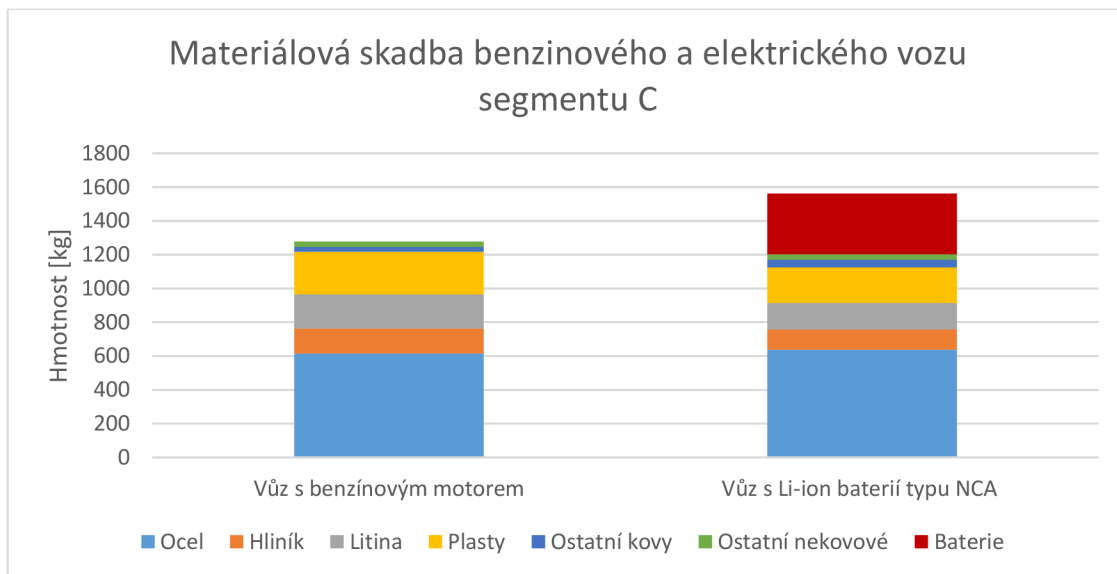
Obrázek 2 Materiálová skladba benzínového a elektrického vozu segmentu C
