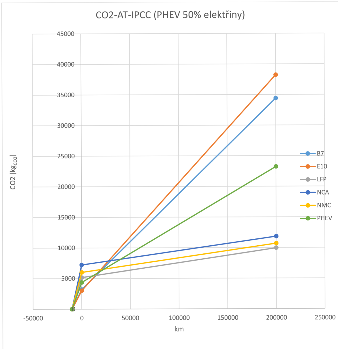
Obrázek 32 CO 2 , Rakousko, metodika IPCC
