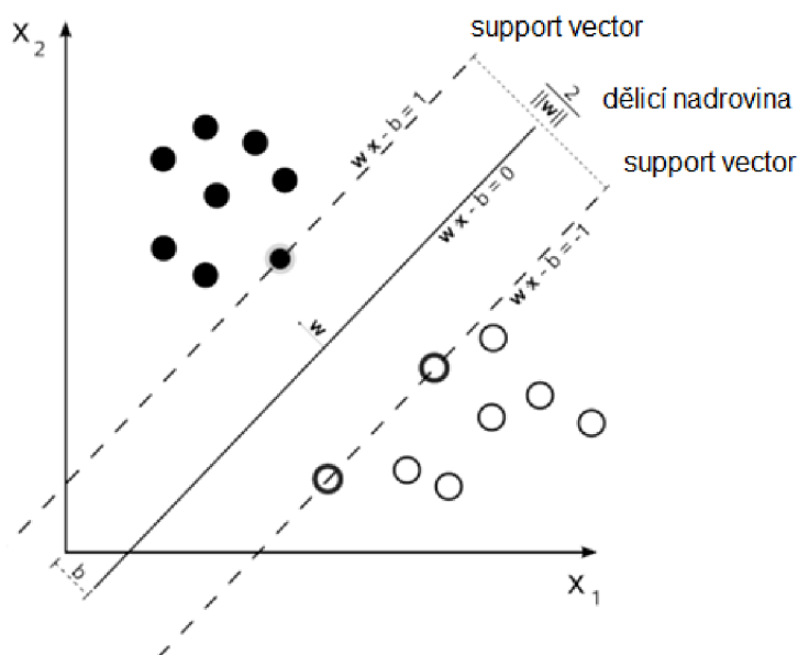
Obrázek 14: SVM rozdělující data do dvou tříd, w – vektor bodů kolmých na oddělující nadrovinu, b – posun nadroviny, x – body (souřadnice) (převzato z [65])
