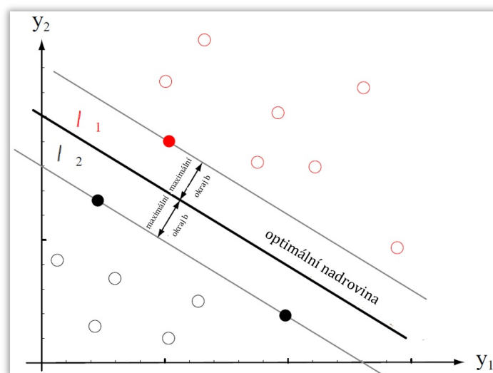
Obrázek 13 – znázornění principu SVM pro 2 třídy, převzato a přeloženo z [14]
