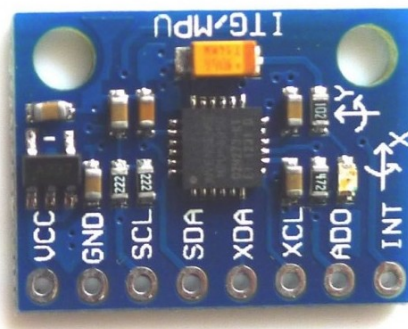
Obrázek 20 – Akcelerometr a gyroskop MCU6050, převzato z [17]
