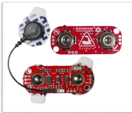
Obrázek 17 – EMG zesilovač MyoWare, převzato z [1]
