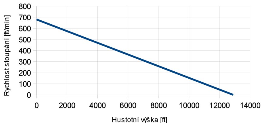
Obr. 3.2.1 – Stoupačí výkon letounu Piper 28 Cherokee, při rychlosti 85 mph a vzletové hmotnosti 2 150 liber.
