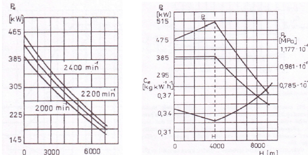
Obr. 3.1.3 – Výškové charakteristiky motoru nasávajícího vzduch (vlevo) a motoru s mechanicky poháněným jednorychlostním dmyhadlem
