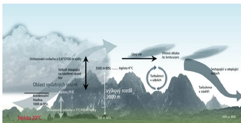
Obr. 4.3.3 - Föhn
