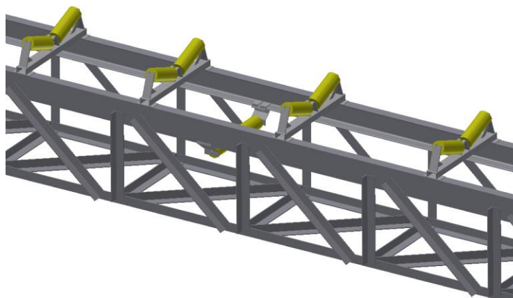
Obr. 24 Rám
