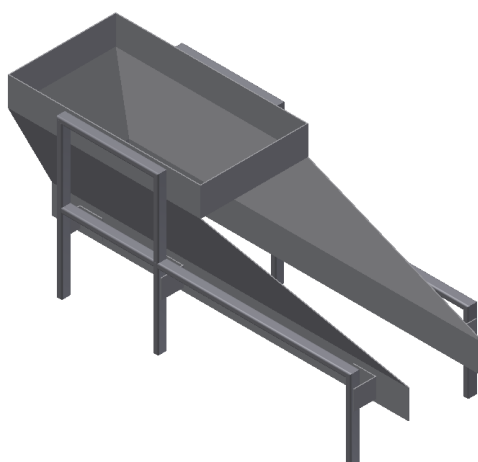
Obr. 27 Násypka
