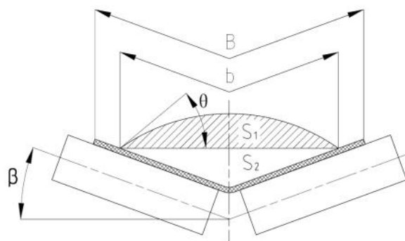
Obr. 9 Šířka pásu
